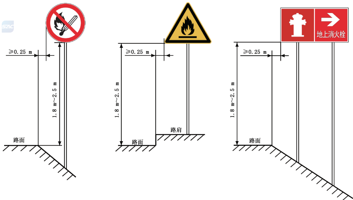
图8 在道路边缘设置的标志牌位置示例
