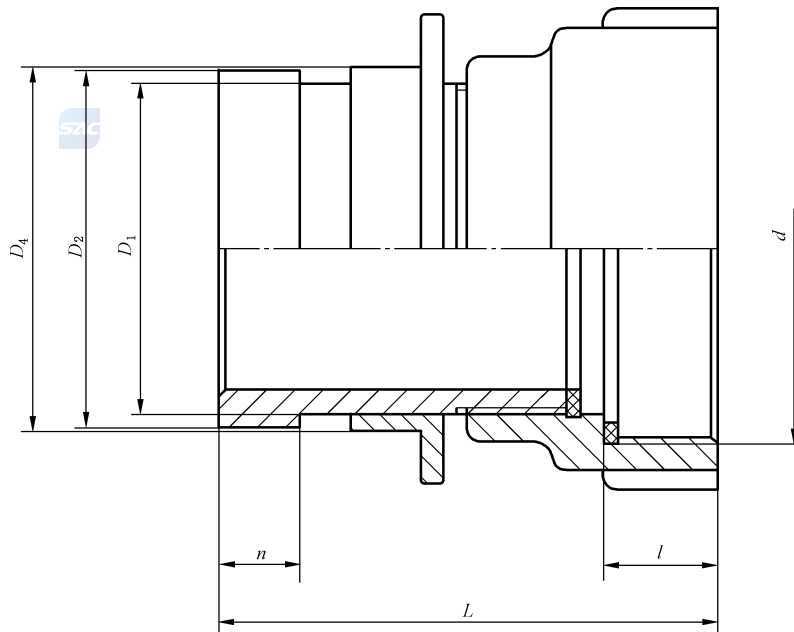
图 B.3 KYKA 型管牙雄接口
