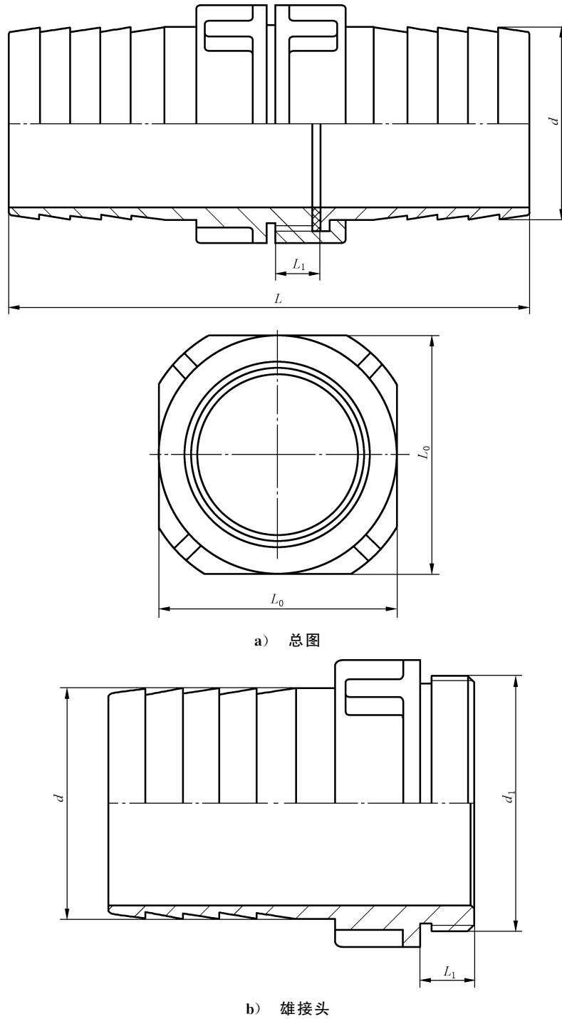
图 C.1 KG 型吸水管接口
