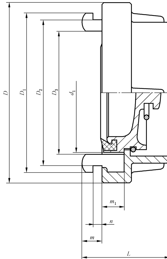
图 A.4 KM 型闷盖
