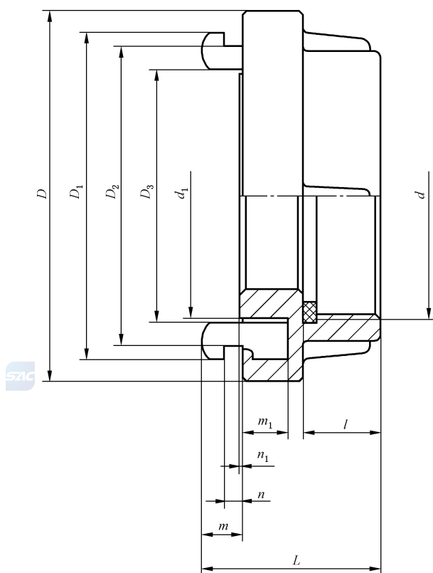
图 A.5 KN 型内螺纹固定接口
