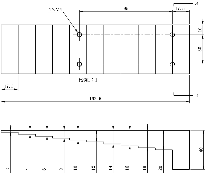
图 A.22 灰度分辨测试物
