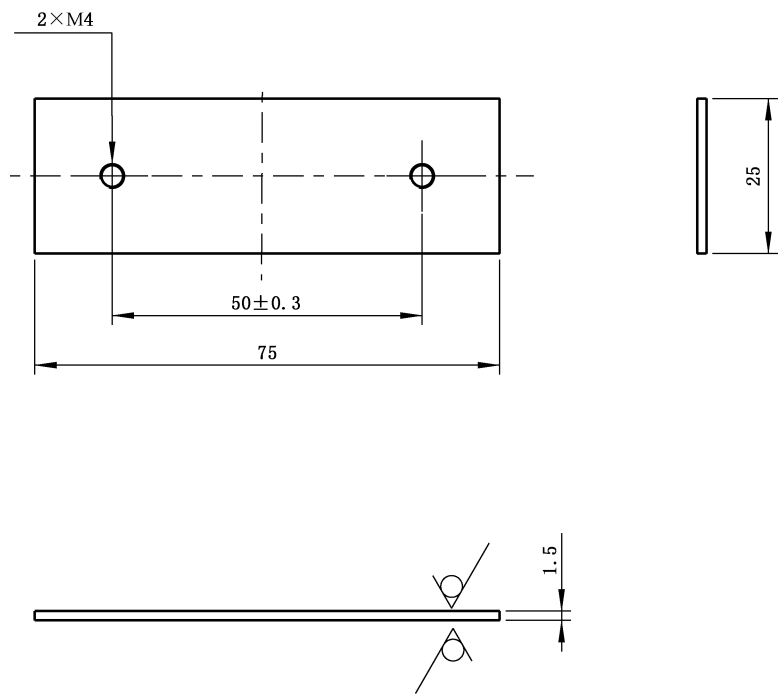
图 A.27 钢板
