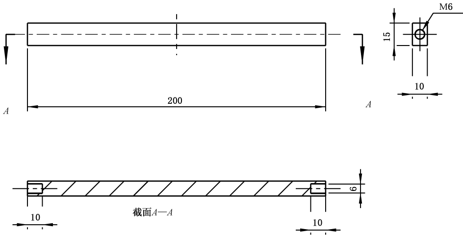
图 A.20 支架横梁
