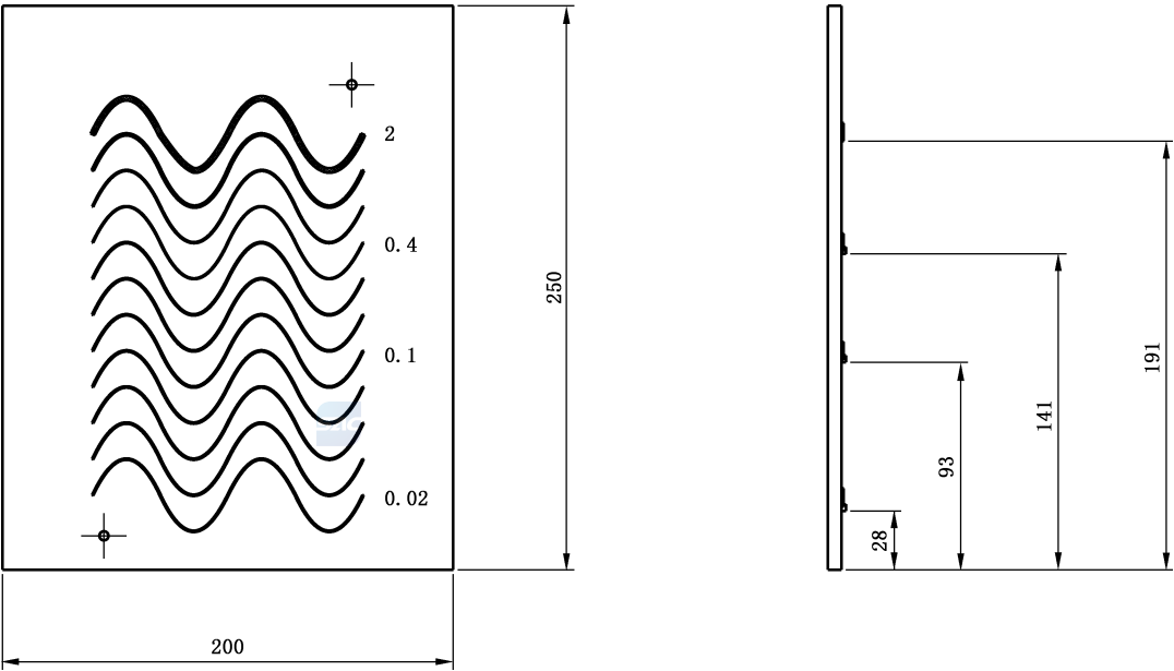
图 A.15 铅字和测试体固定板装配图
