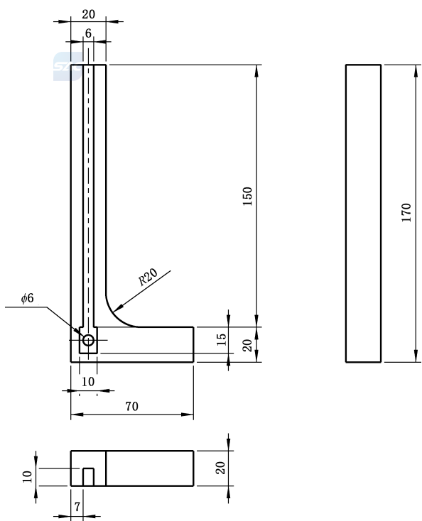
图 A.18 支架 1
