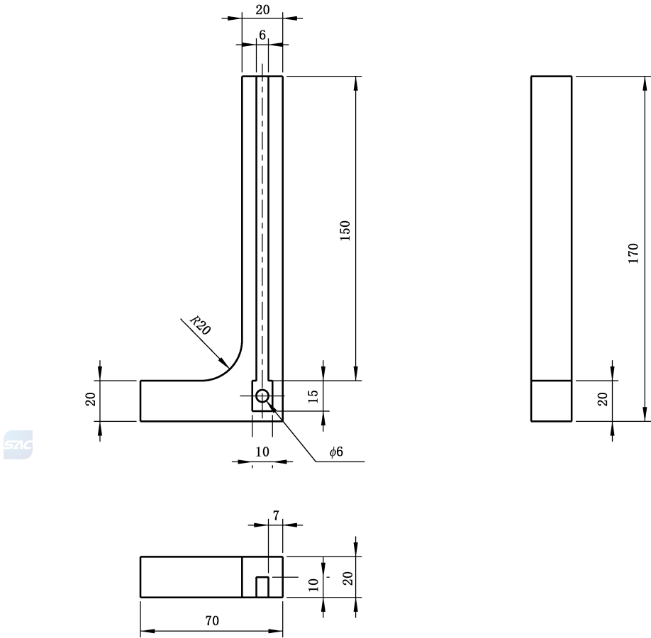
图 A.19 支架 2
