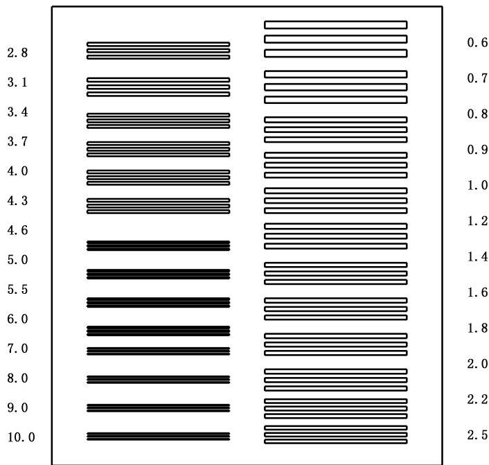
图 A.13 空间分辨力测试卡
