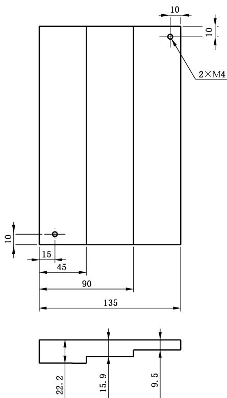
图 A.17 合金铝阶梯
