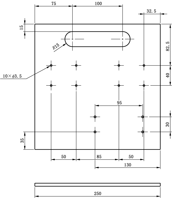
图 A.23 测试物固定板
