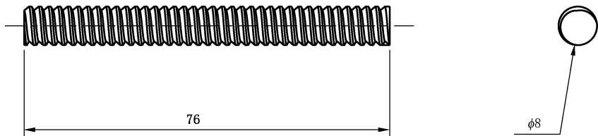
图 A.8 短螺杆
