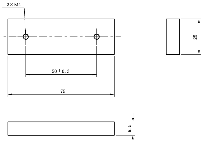
图 A.26 PVC 板
