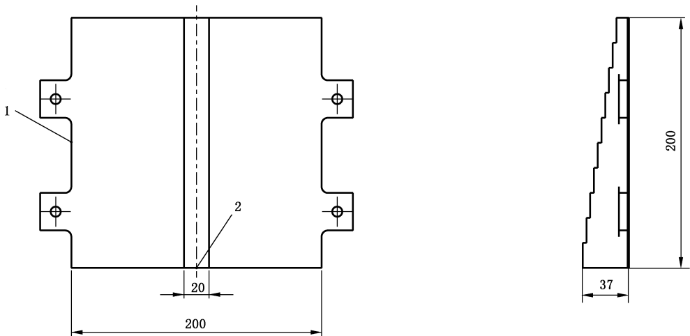
图 A.1 穿透力测试体
