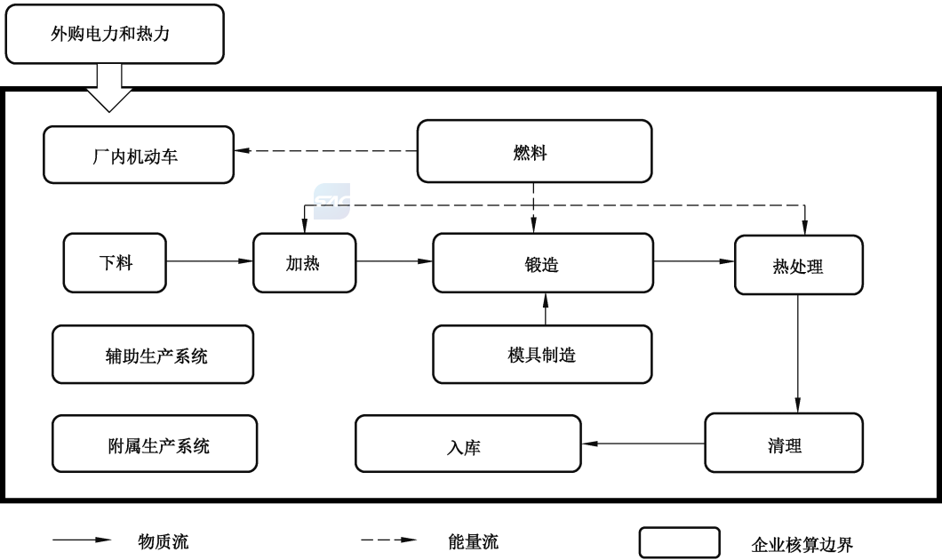
图 A.1 锻造企业碳核算边界示意图
