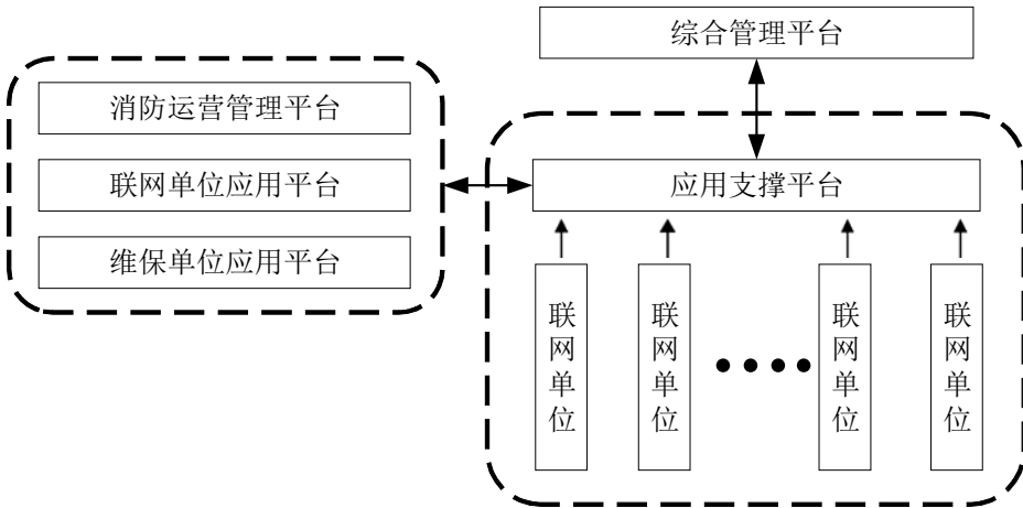
图2 消防物联网系统的网络连接图
