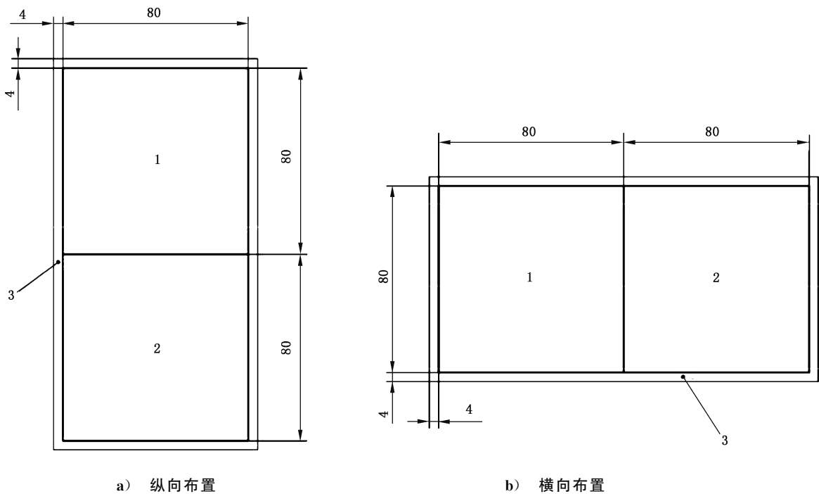
标引序号说明： 1——含有安全警告符号或以安全警告三角形为边框的描述危险图示的图示框； 2——含有避免危险图示的图示框； 3——边框。 机器安全标签的圆角可有一个与标签的尺寸成比例的小半径。可以根据安全标志的尺寸、背景对比和可视清晰度，对边框宽度进行调整。
