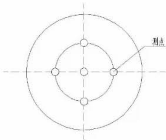
图 4 圆形风口测点布置
