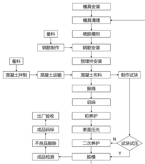
图 6.2.1 预制混凝土构件基本生产工艺流程
