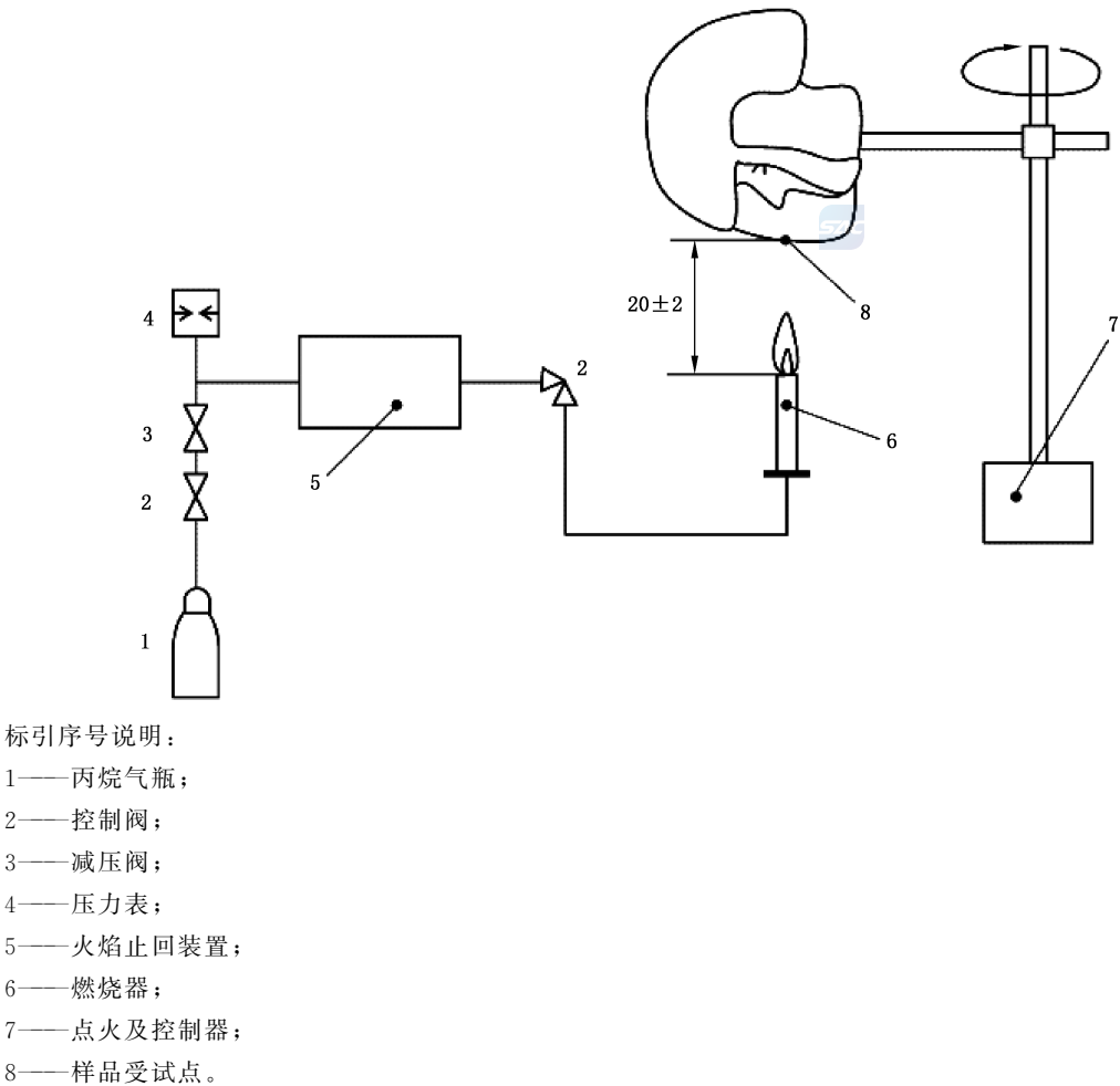
图 11 可燃性测试装置示意图
