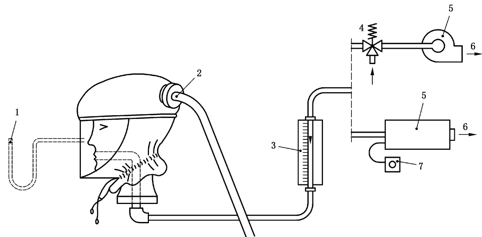
图 9 开放型面罩送气量测试装置示意图
