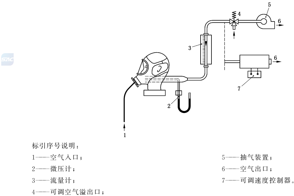
图 8 密合型面罩送气量测试装置示意图
