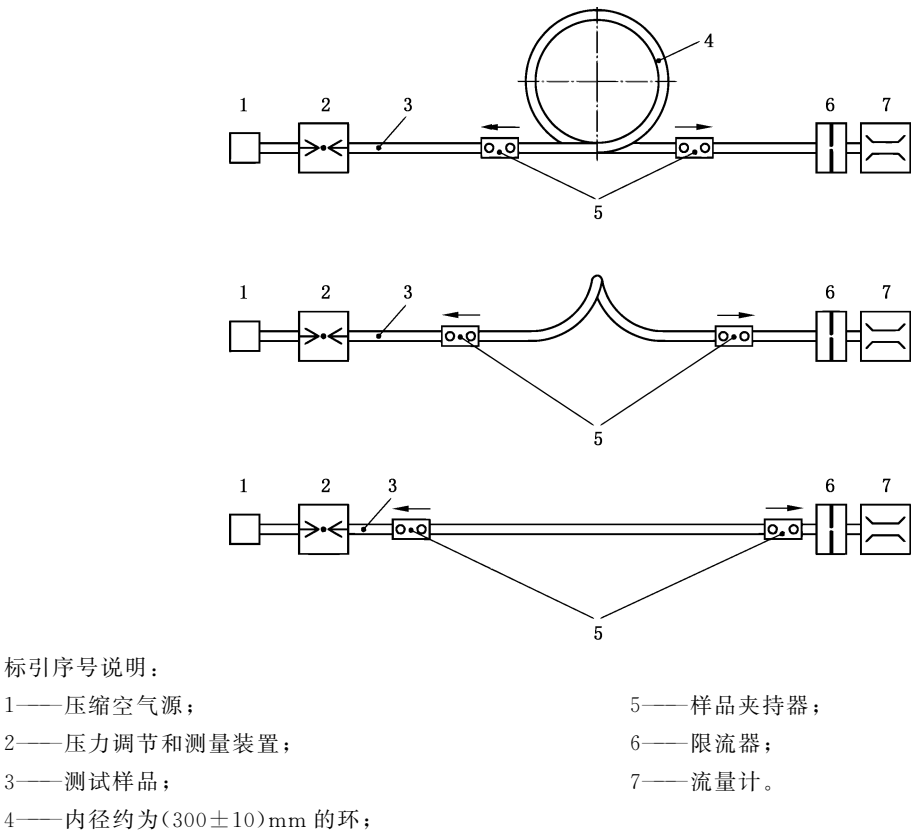
图 6 逆时针方向旋转时中压送气管抗扭结性的检测过程示意图
