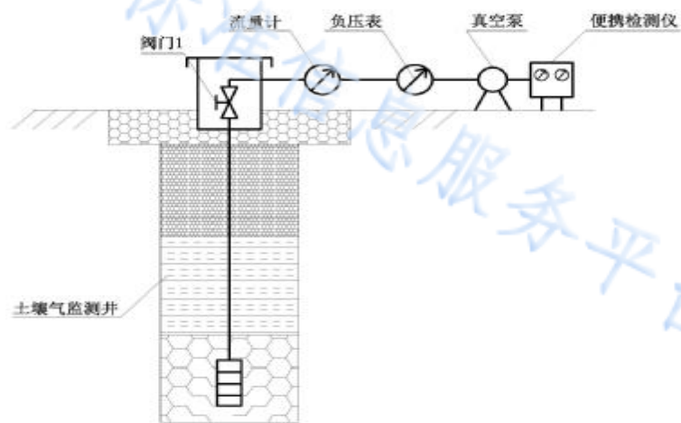
图4 洗井系统示意图
