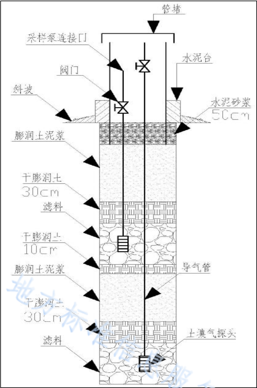
图F.1 土壤气监测井结构图
