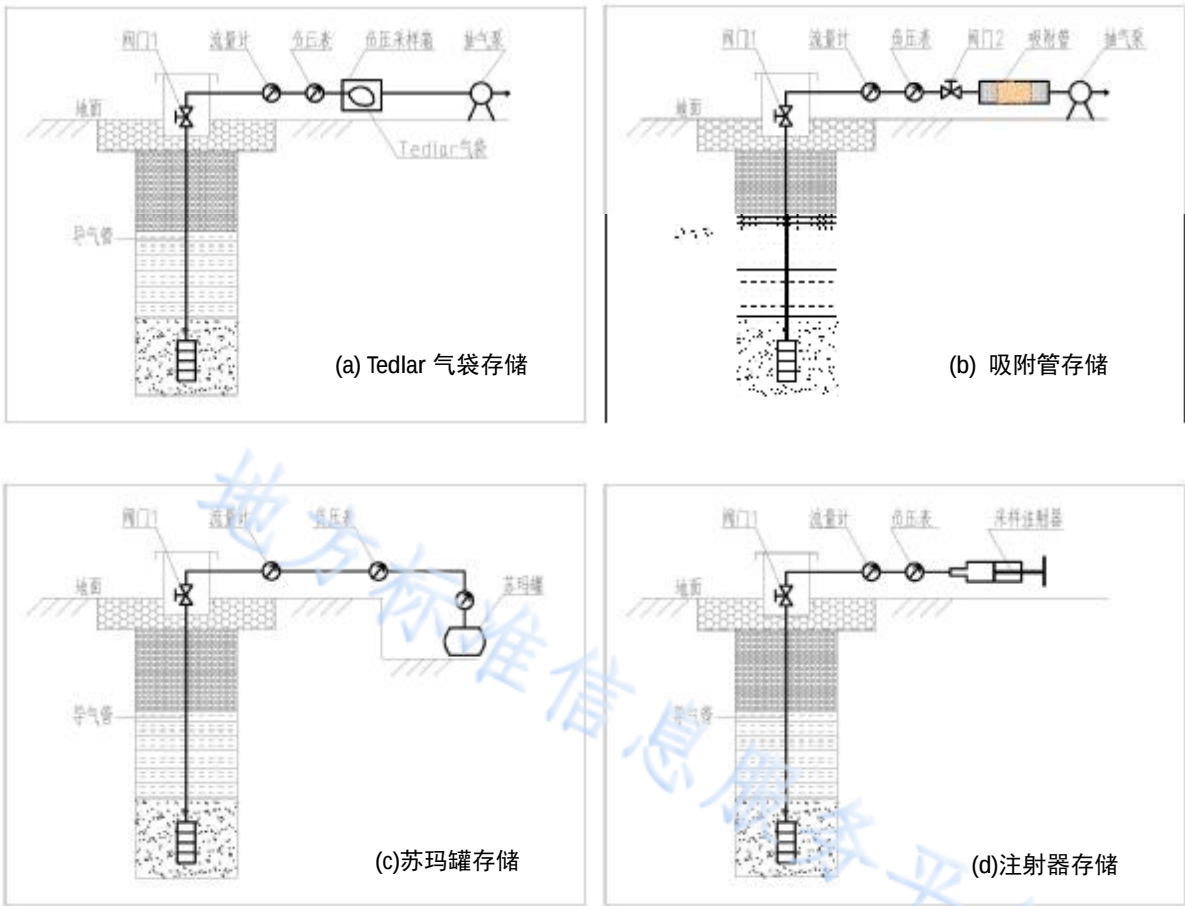
图 I.3 不同样品存储设备采样系统连接示意图
