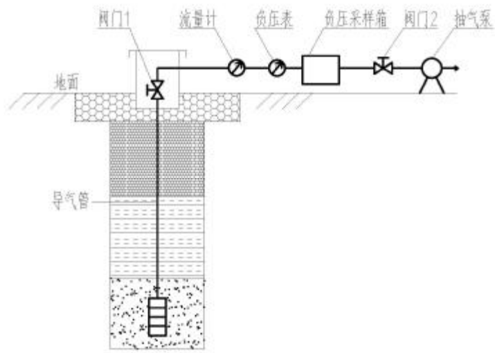
图3 采样系统渗漏监测系统示意图
