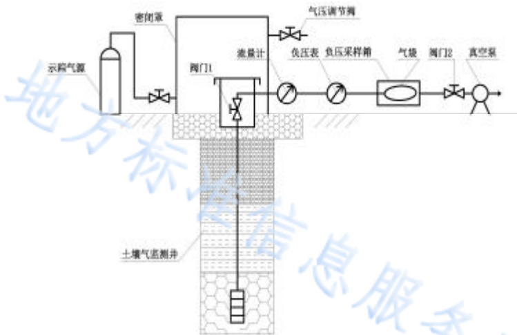
图2 土壤气监测井气密性测试示意图
