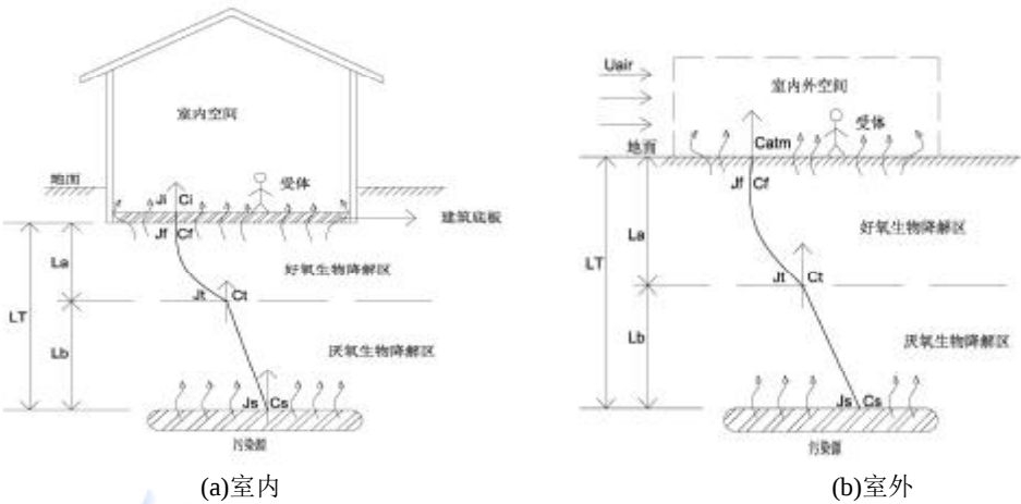
图 J.1 挥发性有机物迁移概念模型
