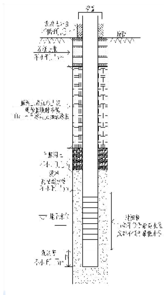
图D.1 地下水监测井结构图
