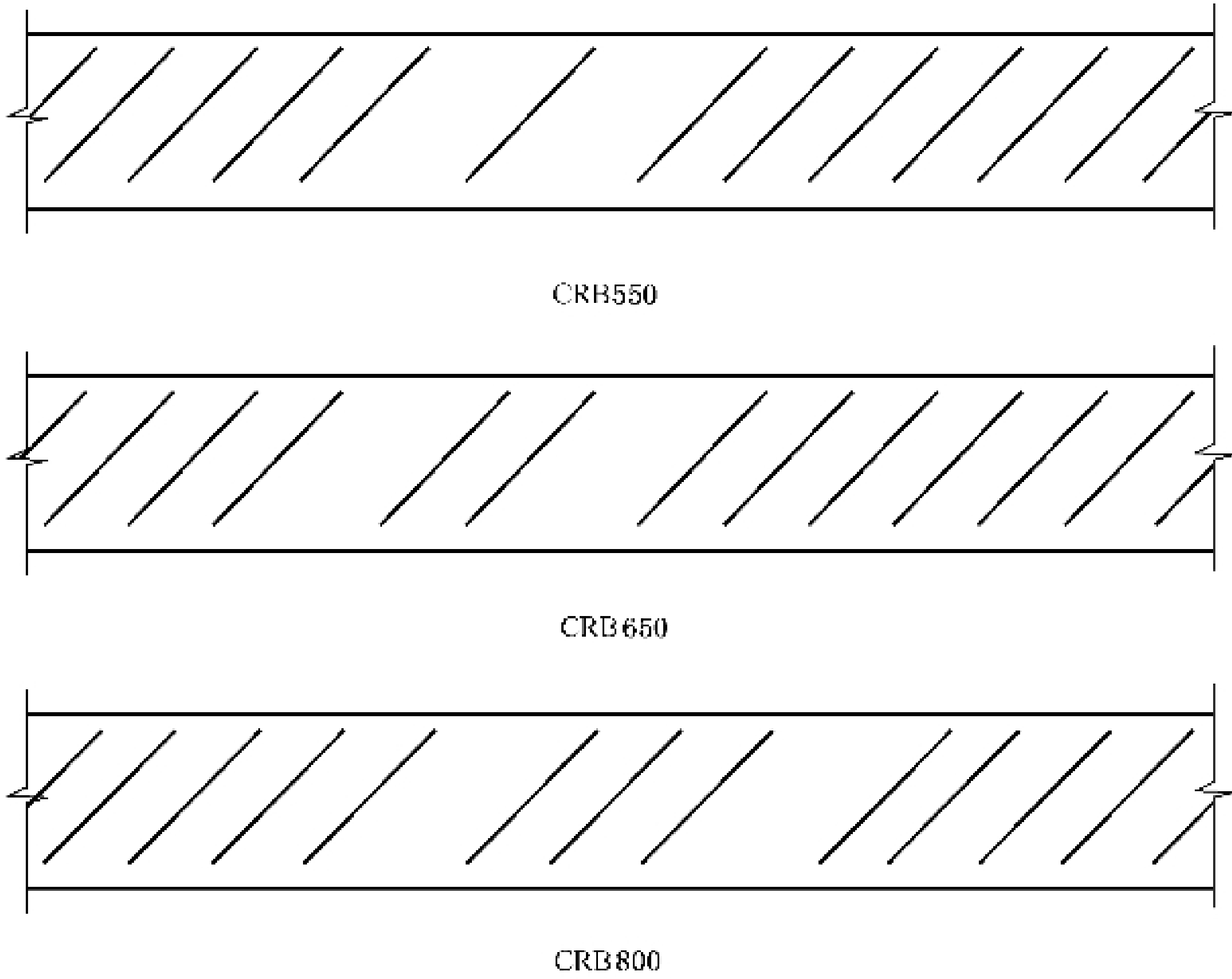
图 3 冷轧带肋钢筋标志示例
