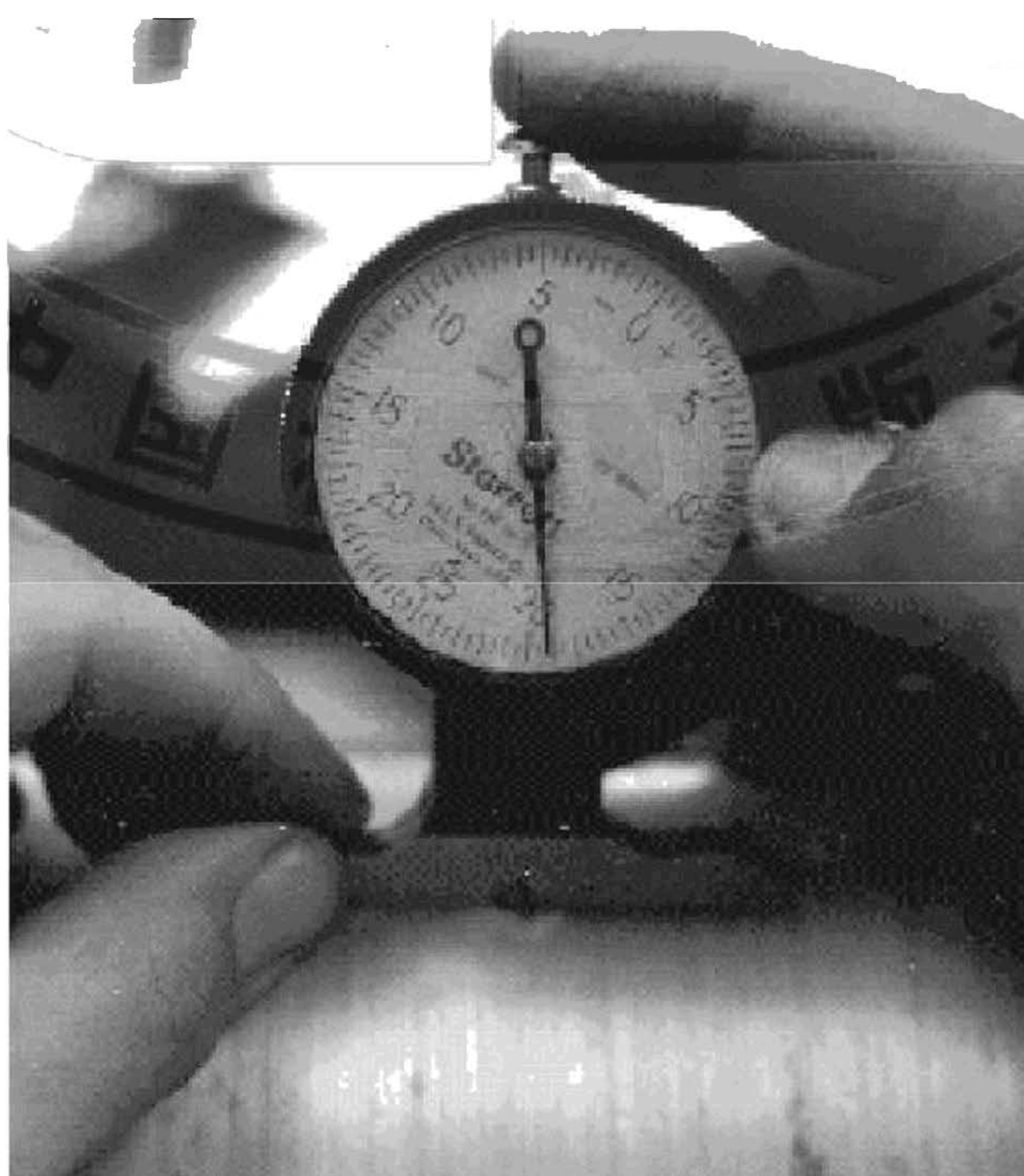
图 F.13 深度测量
