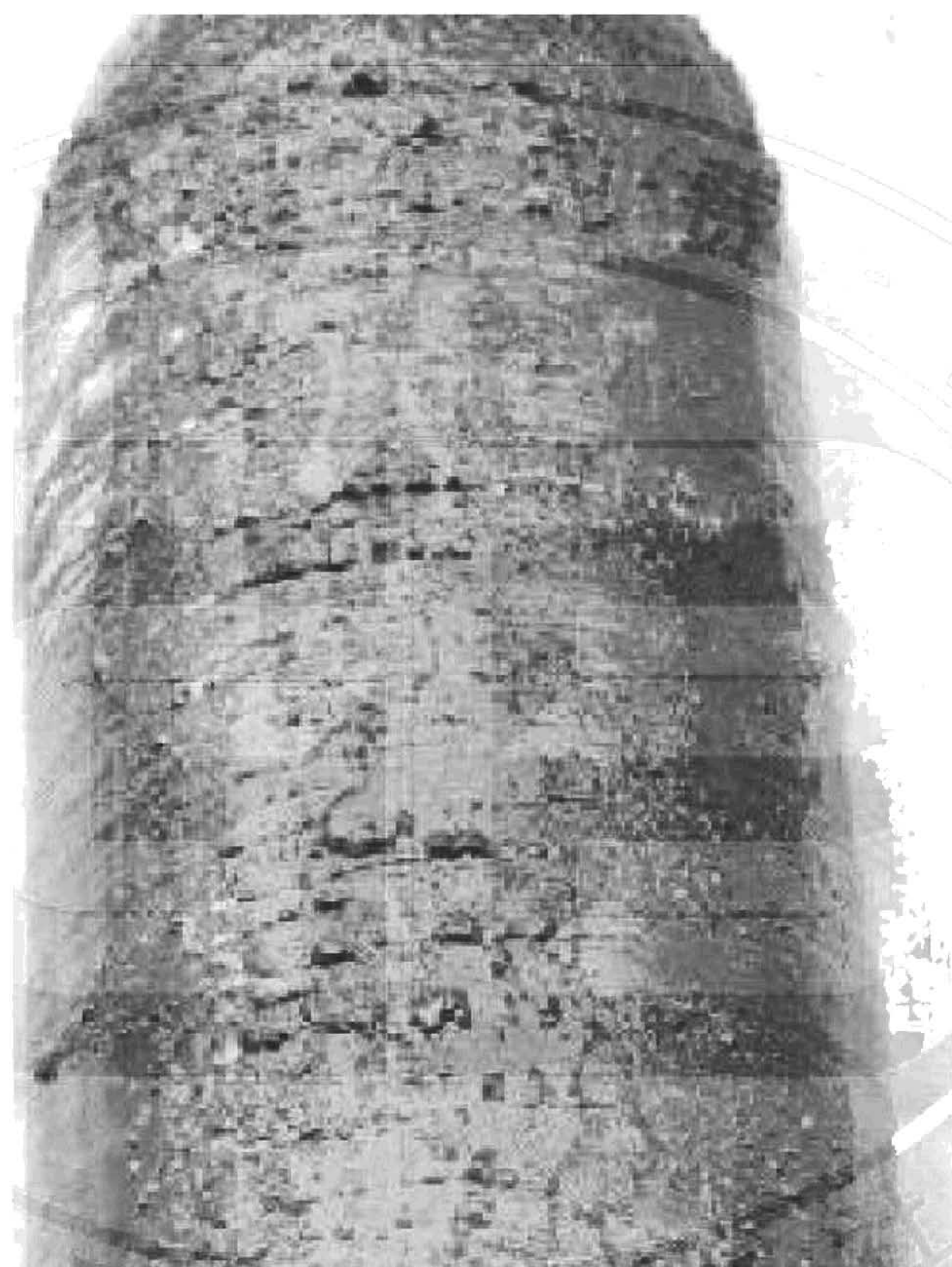
图 F.1 化学品腐蚀(报废)
