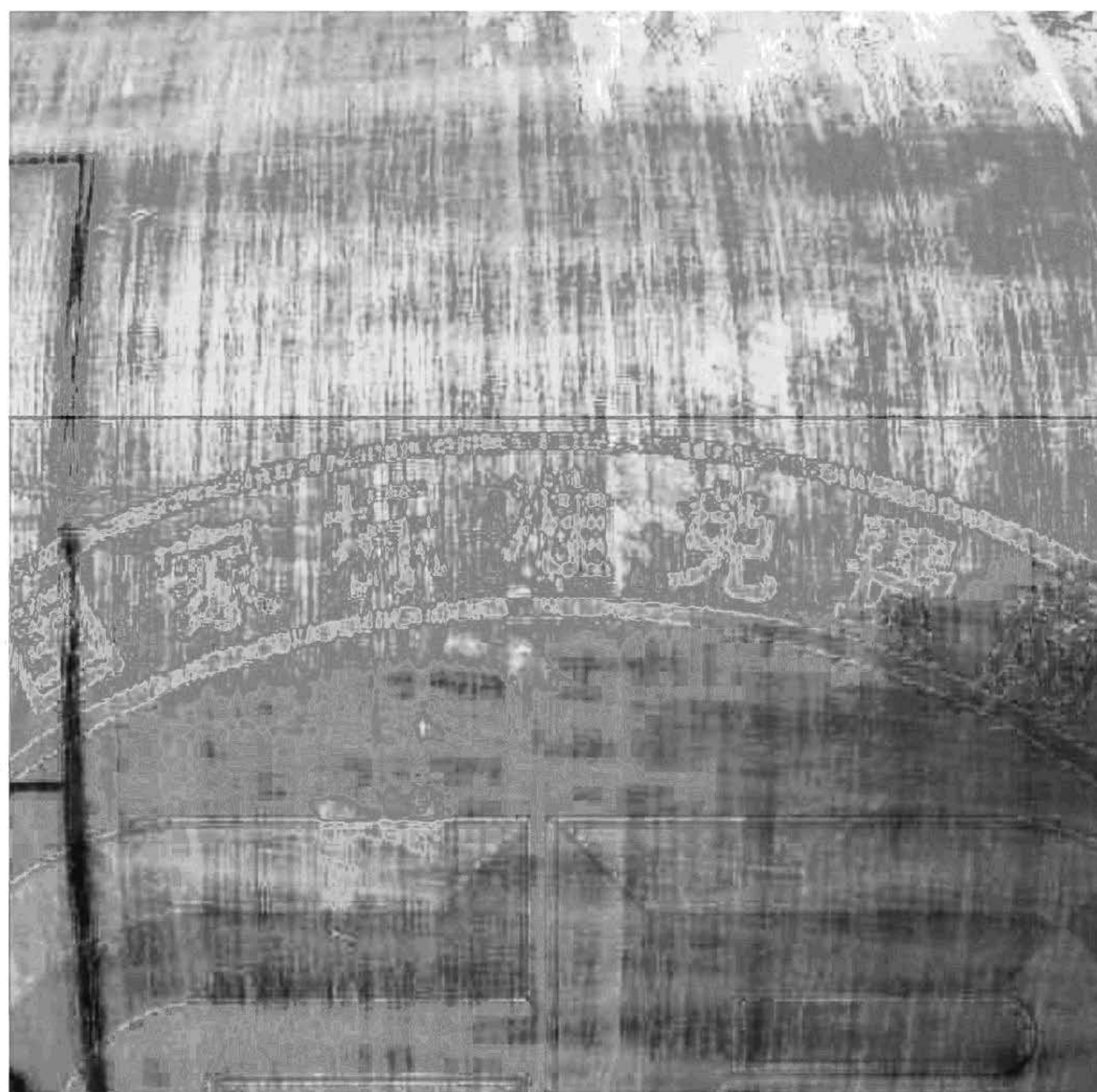
图 F.2 一级磨损(允许的)
