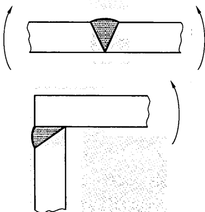
图 B. 4b) 不允许的例子(或在 6.2 规定安全系数提高 50%的情况下允许)
