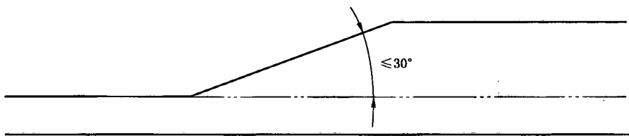
图 B. 1 壁厚突然改变
