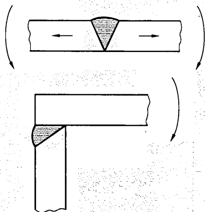
图 B. 4a) 允许的例子
