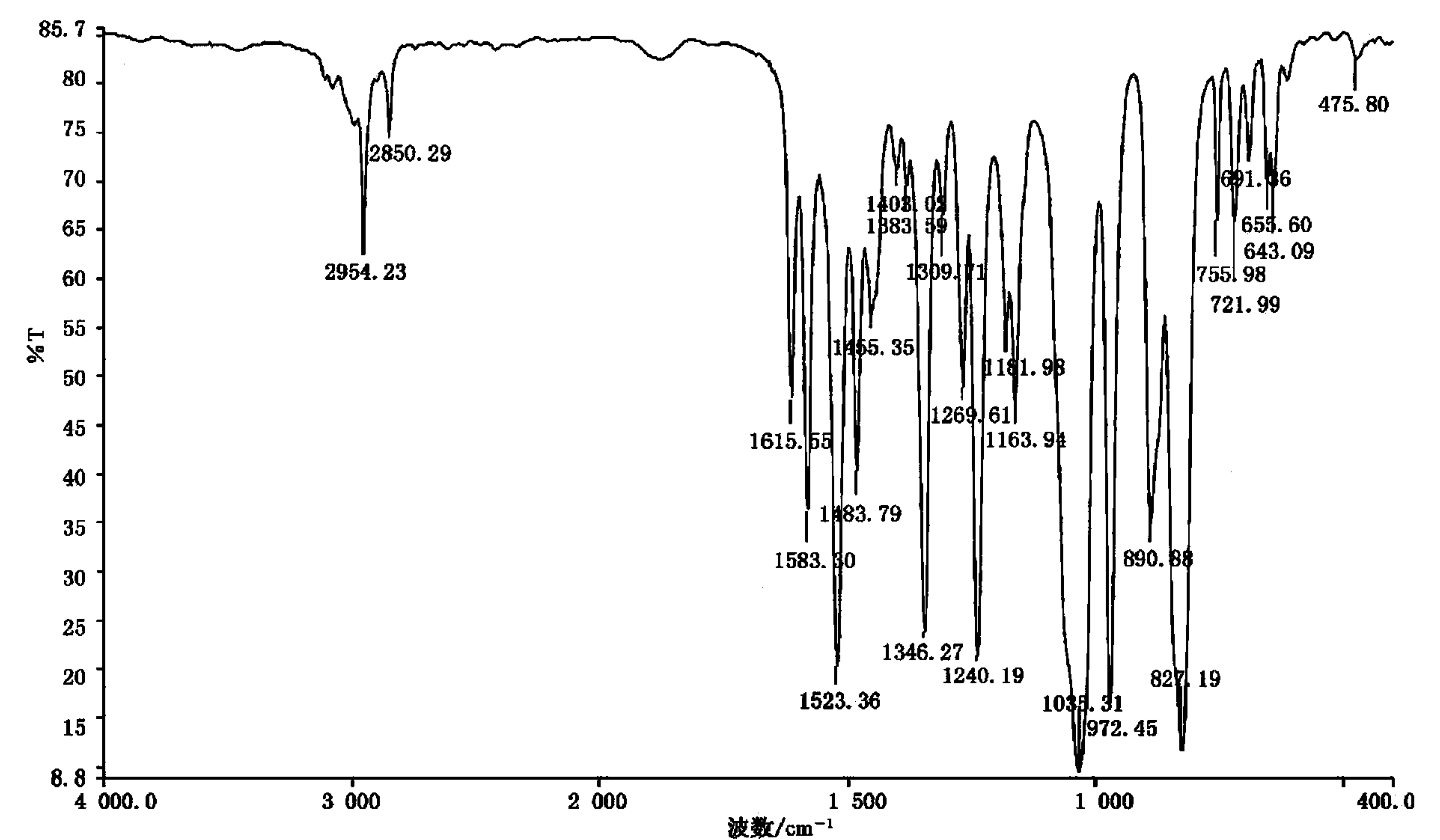
图 1 杀螟硫磷标样的红外光谱图
