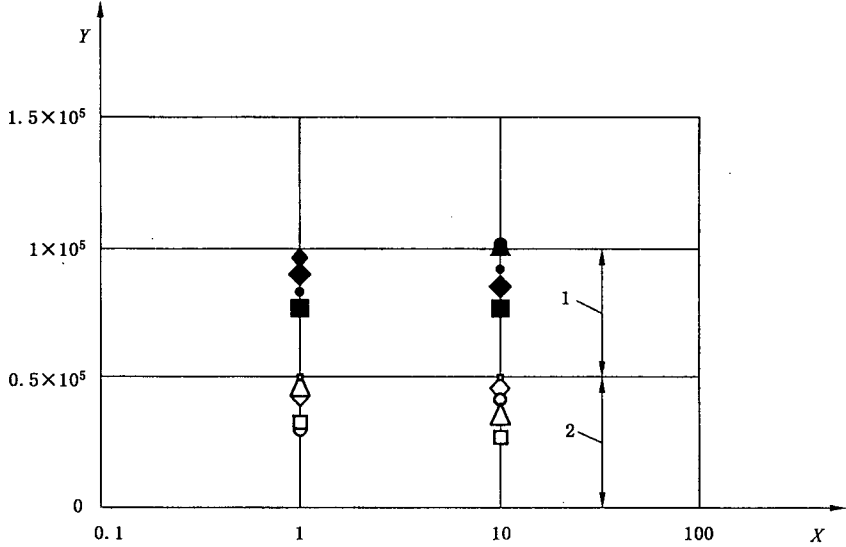
图解: 1——范围 2: 对于 p = p_{red,max} = 1 \times 10^5 \text{ Pa} , N = C_2 \times V_{2/3} ; 2——范围 1: 对于 p = p_{red,max} = 0.5 \times 10^5 \text{ Pa} , N = C_1 \times V_{2/3} ; Y—— p_{red,max} , 单位: Pa; X——容器容积 V , 单位: \text{m}^3 。
