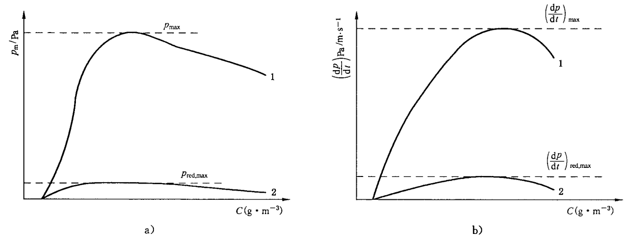
图例： 1——未抑制的爆炸； 2——抑制的爆炸。 注：触发压力 p_a 与抑制器数量(抑制物荷载)不变。
