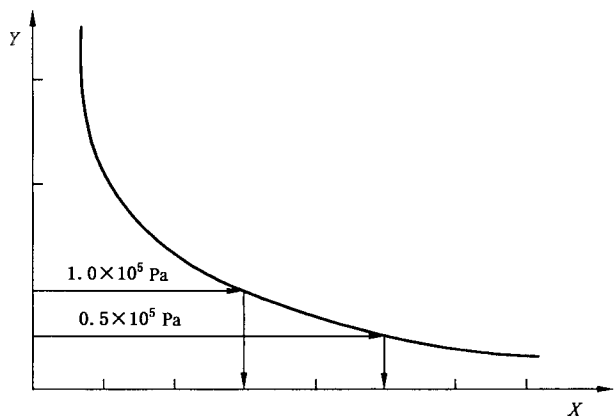
图解 X——HRDs; Y—— p_{\text{red,max}} (Pa)。 注：爆炸常量 K_{\text{max}} 和触发压力 p_a 不变。
