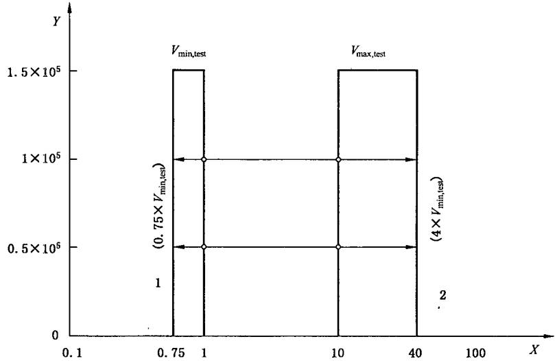
图解: 1——外壳容积下限; 2——外壳容积上限; Y—— p_{red,max} , 单位: Pa; X——容器容积 V , 单位: \text{m}^3 。
