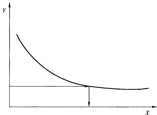
图解: X—— p_s (Pa); Y—— p_{\text{red,max}} (Pa)。 注：触发压力 p_a , 爆炸常量 K_{\text{max}} 及 HRD 抑制器的数目不变。
