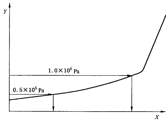
图解 X —— K_{max} ( \text{m}\times\text{Pa}/\text{s} ) ; Y —— p_{red,max} (Pa)。 注：触发压力 p_a 与 HRD 抑制器数量(抑制物荷载)不变。
