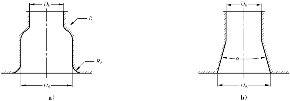
图 4 爆破试验装置与爆破片安全装置连接变径管内部轮廓的示意图
