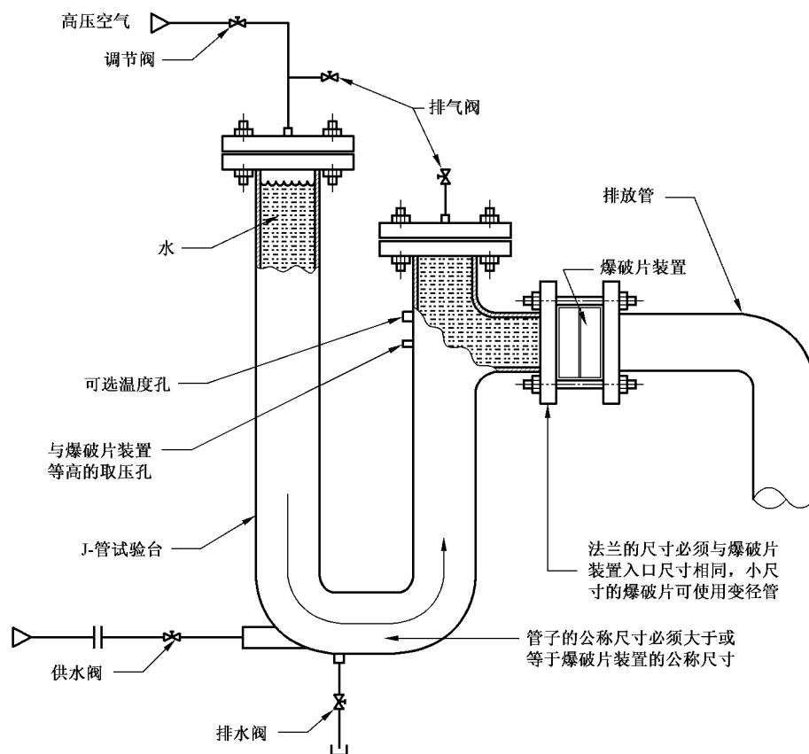
图 2 使用液体介质的爆破片爆破试验装置示意图
