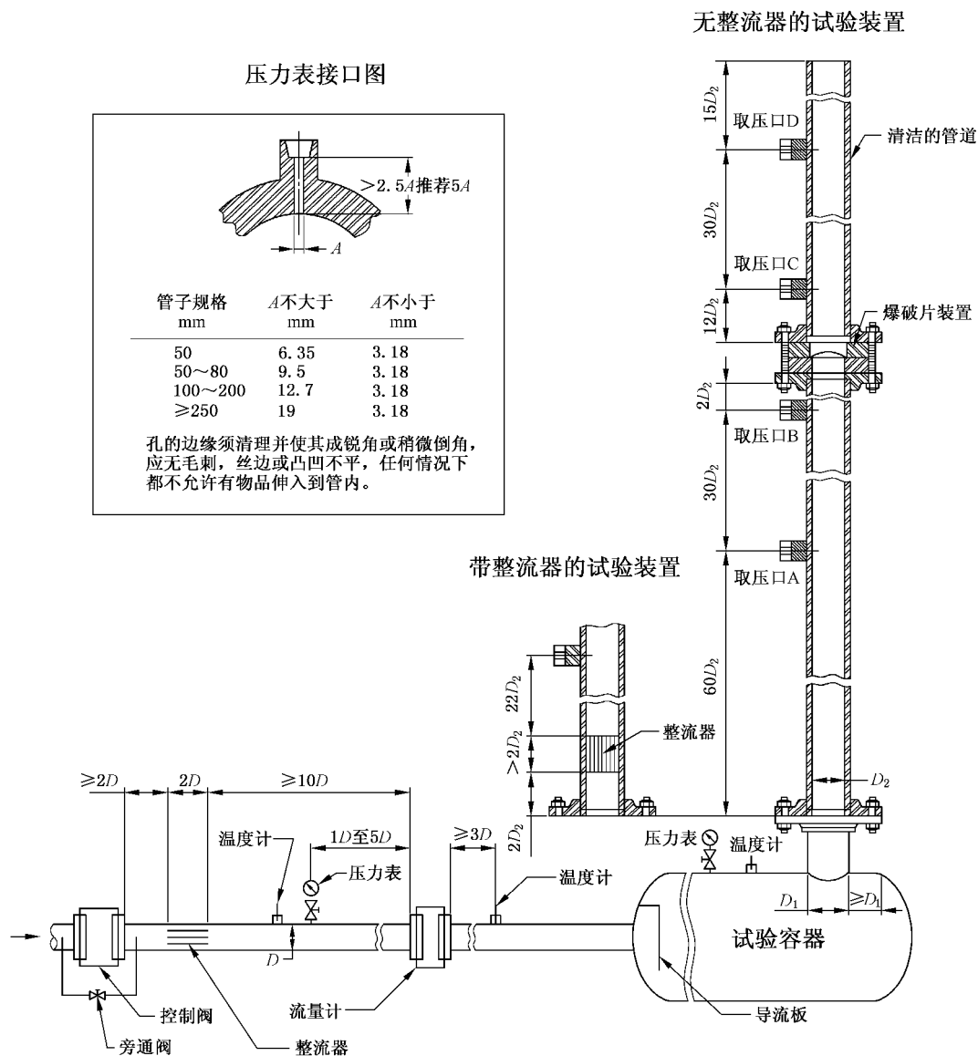
图 5 爆破片安全装置流阻试验装置示意图
