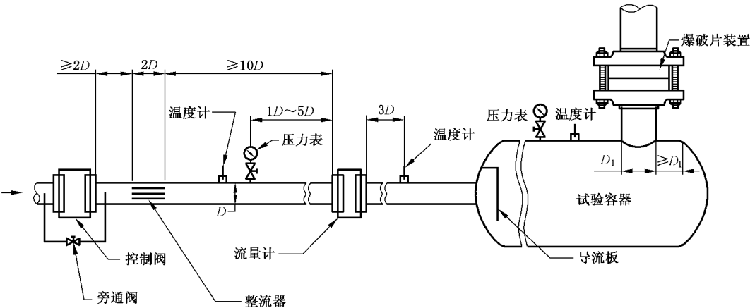
图 3 泄放量试验装置示意图
