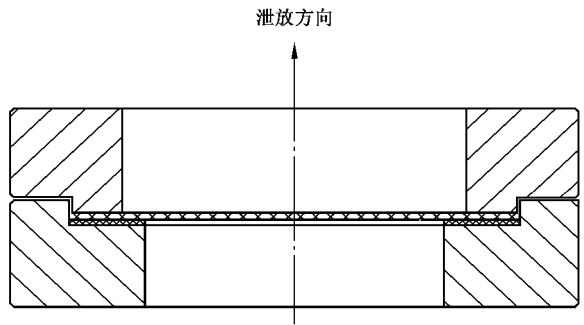
图 9 单片可更换型石墨爆破片夹持器
