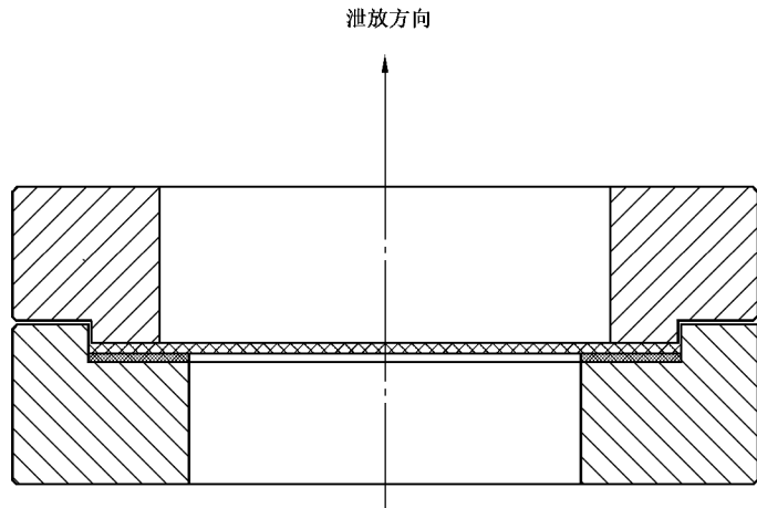
图 4 石墨爆破片
