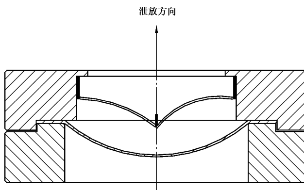
图 7 反拱刀架型爆破片夹持器
