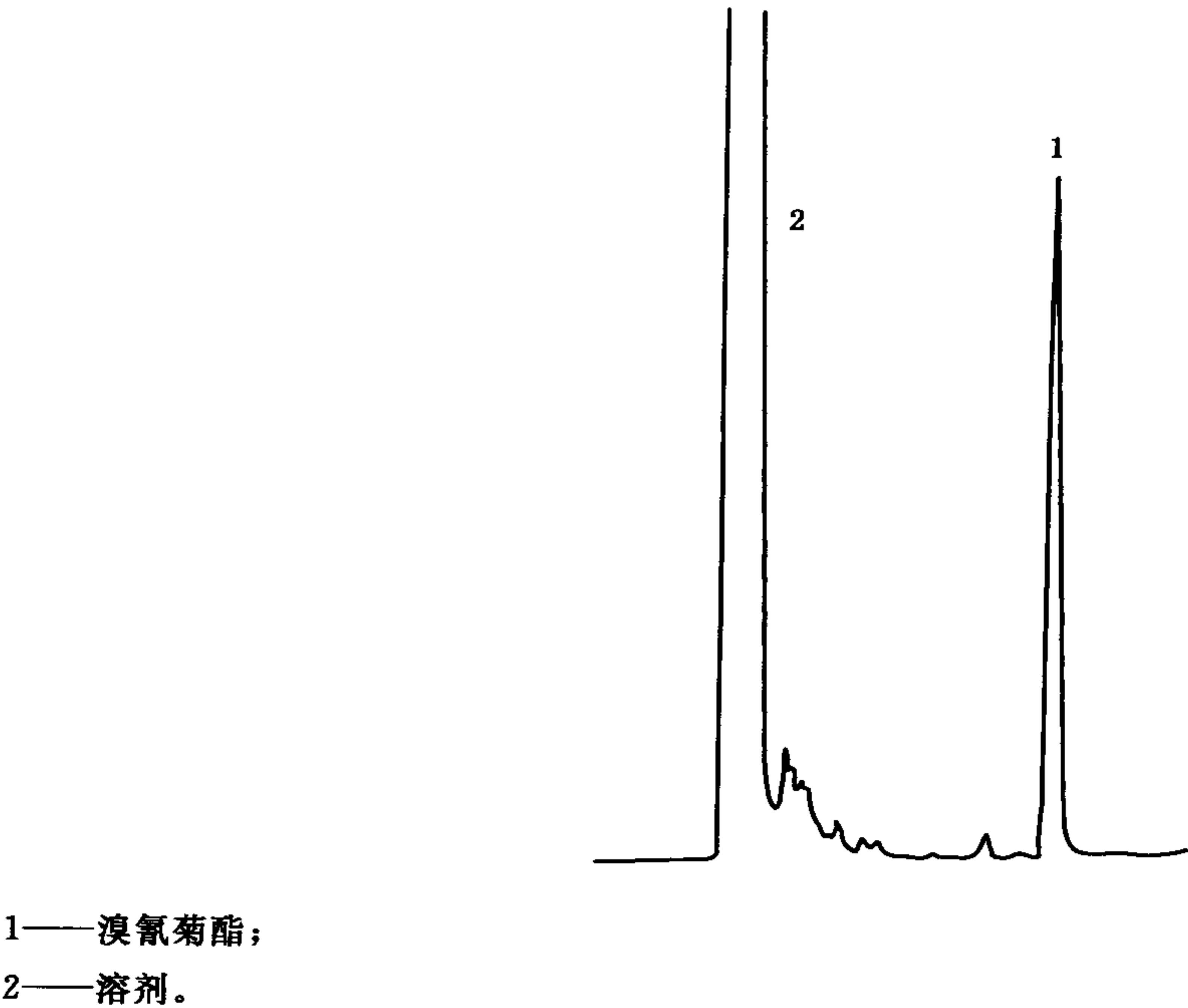
图 1 溴氰菊酯乳油的正相高效液相色谱图
