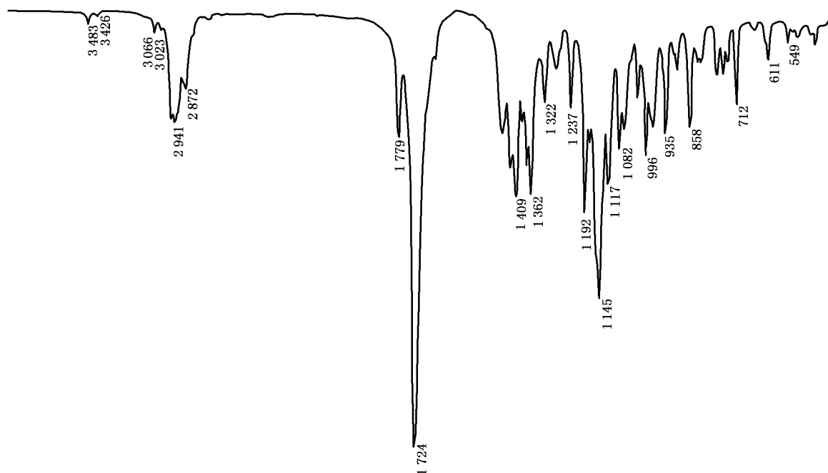
图 1 胺菊酯标样的红外光谱图
