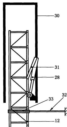
c) 外爬升
