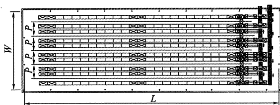
图 B. 0. 3-1 自动化库平面
