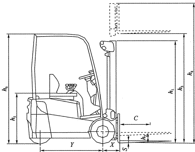
图 A.0.1-1 叉车立面
