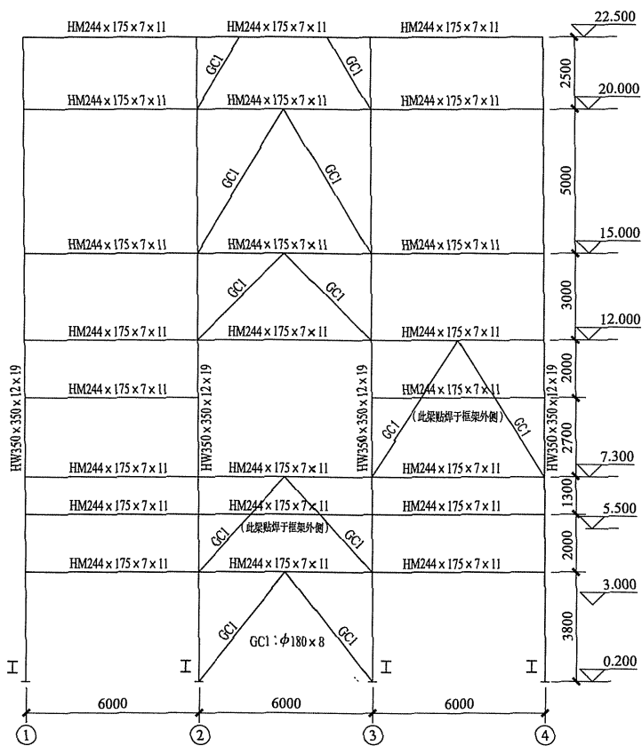
图 10 SS-4④轴线立面
