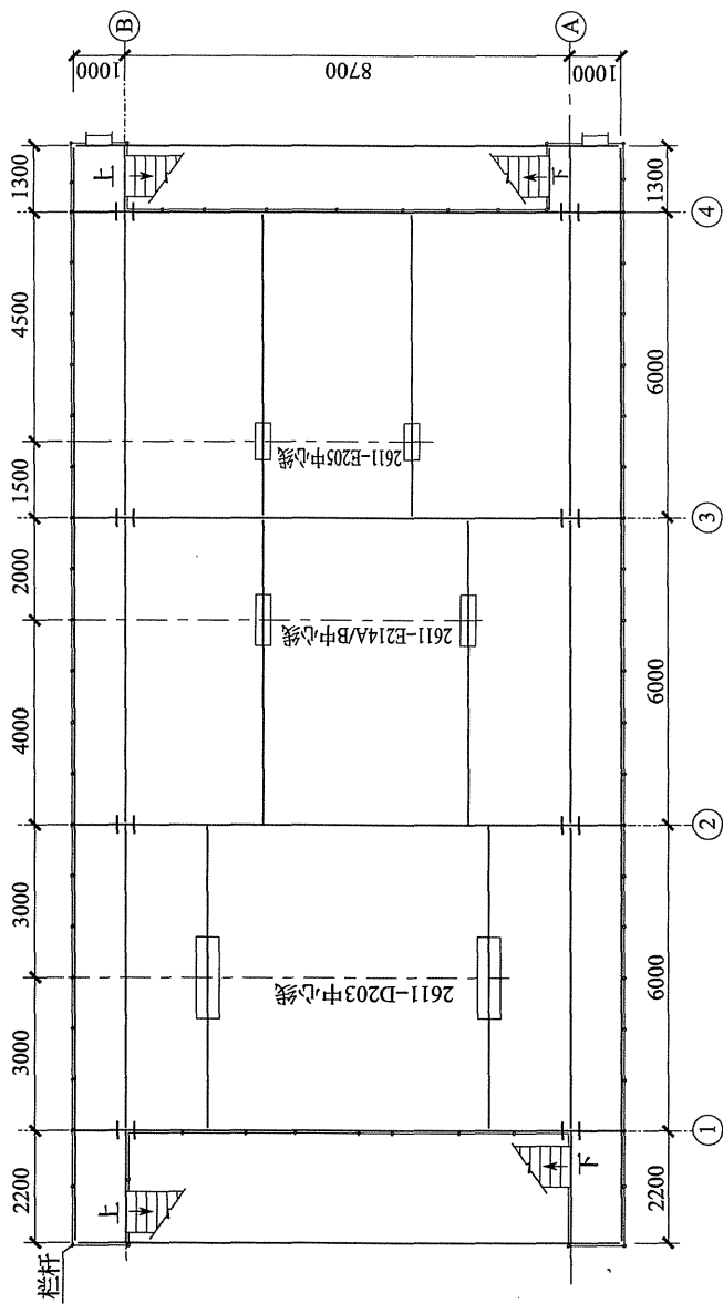
图 6 SS-4 标高 7.30m 平台
