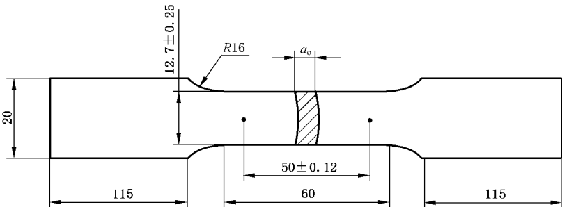
图 3 拉伸试样
