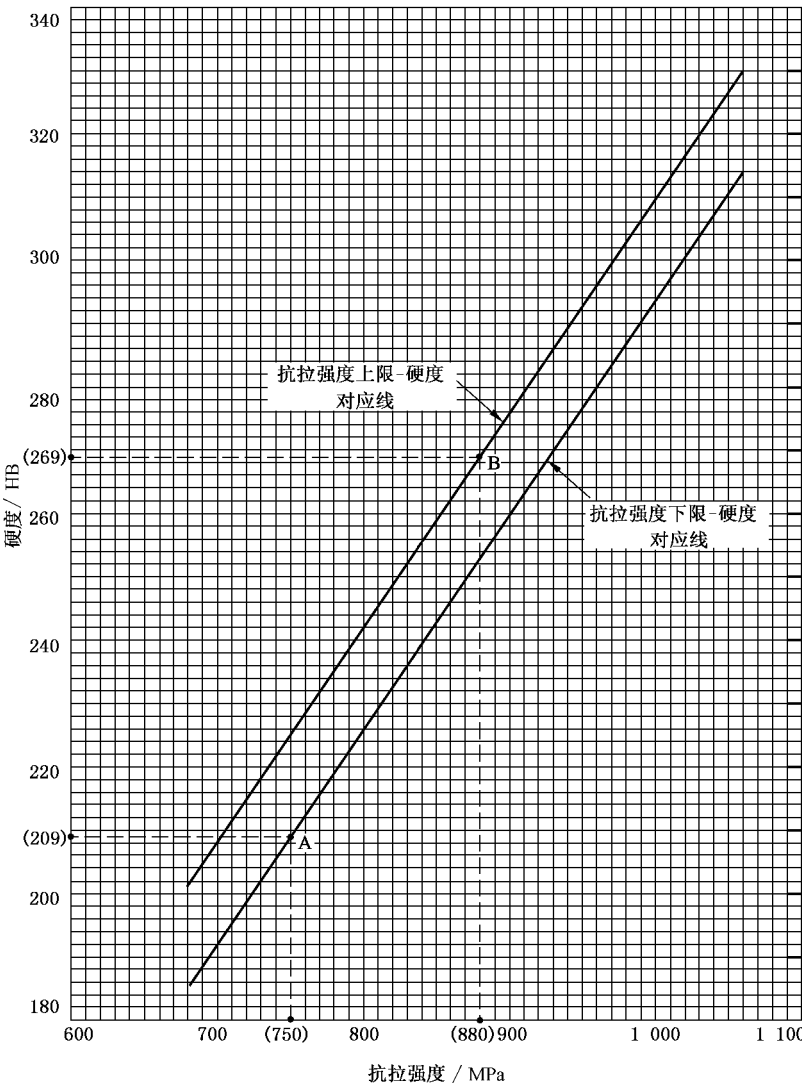
图 E.1 硬度-抗拉强度对应图
