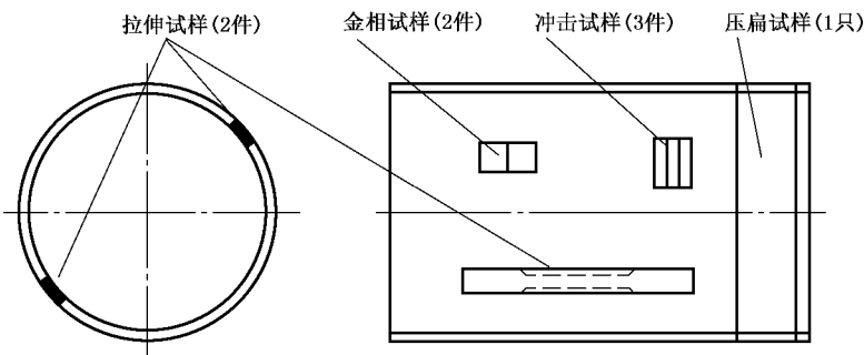
图 2 取样部位图
