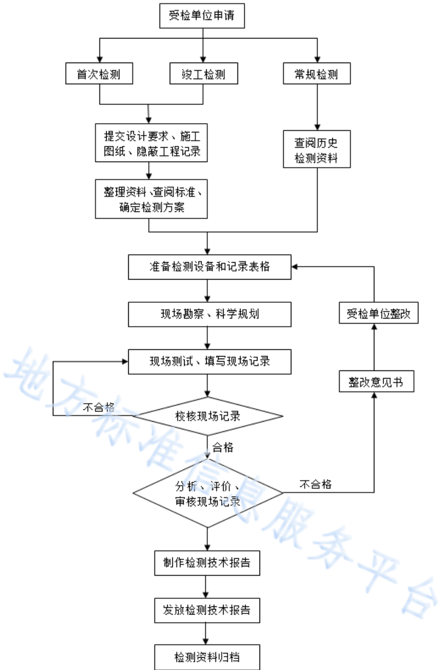
图A.1 地铁系统防雷装置检测程序流程图
