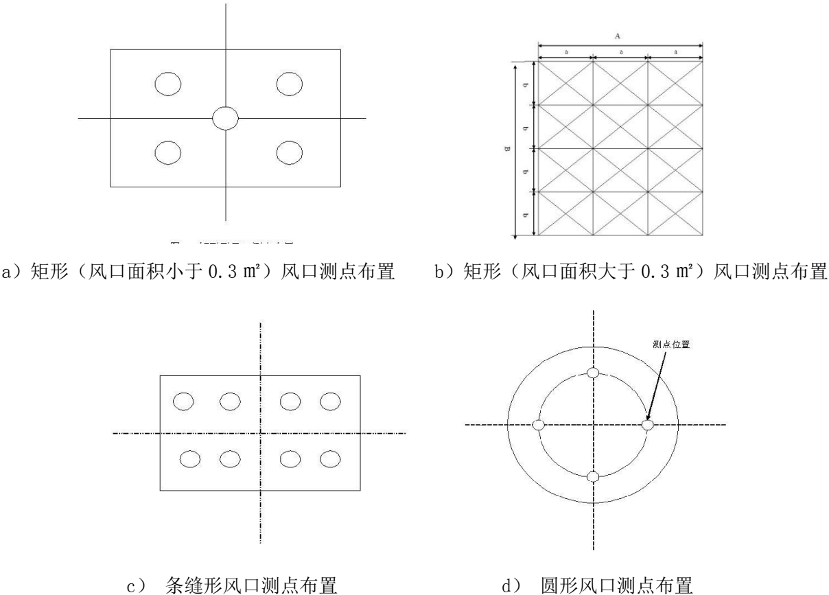
图1 不同形状风口测点布置
