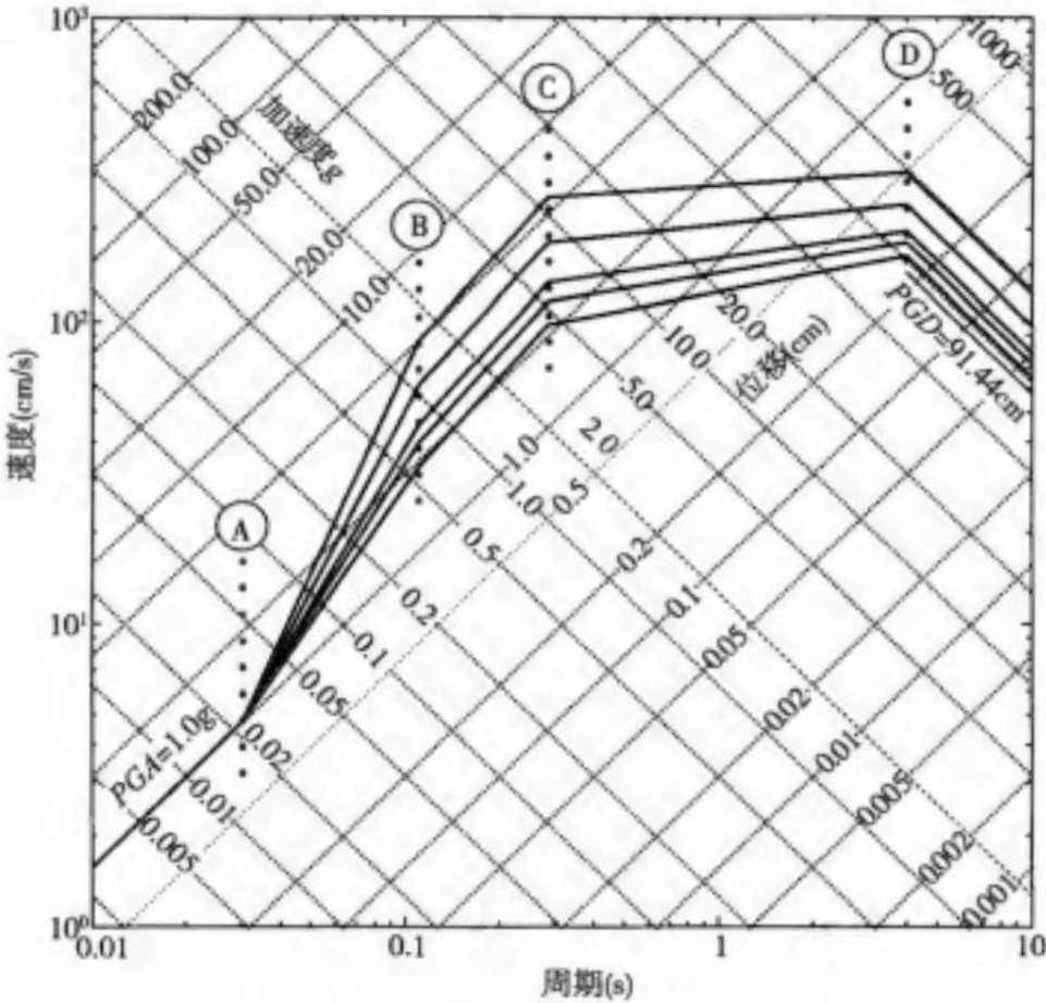
图 F.0.2 竖向反应谱
