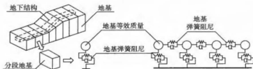
图 3 地震动计算模型
