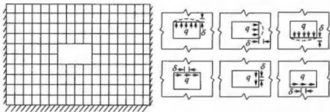
图 2 地基等效弹簧刚度的计算
