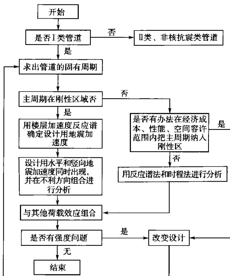
图5 I类管道抗震设计流程图
