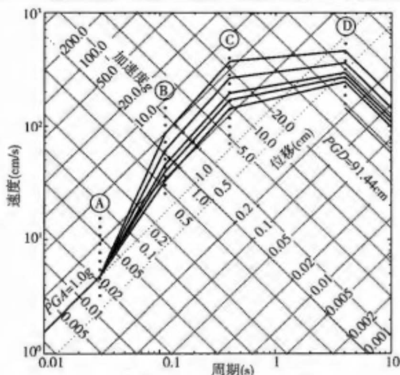
图 F.0.1 水平向反应谱
