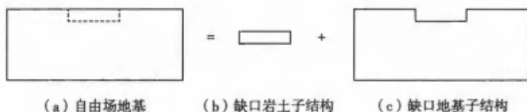
图 A. 3. 2 自由场地基模型示意图
