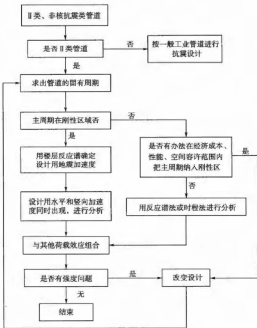
图 6 非 I 类管道抗震设计流程图
