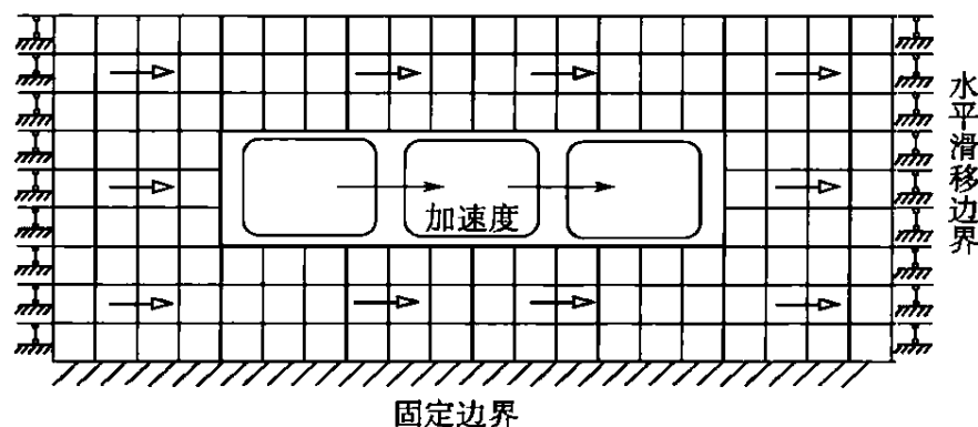
图 J.2.1 反应加速度法计算模型示意图
