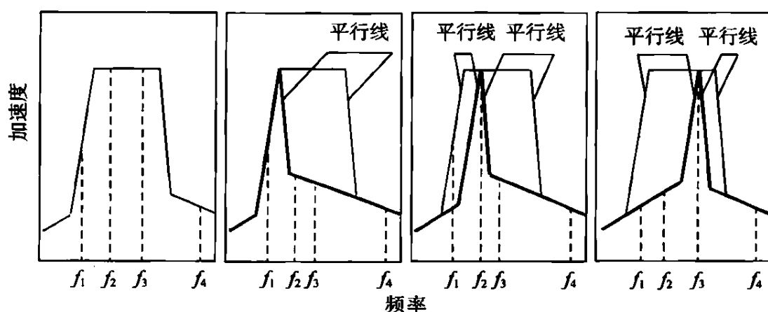
图 D.0.4 楼层反应谱的调整示例
