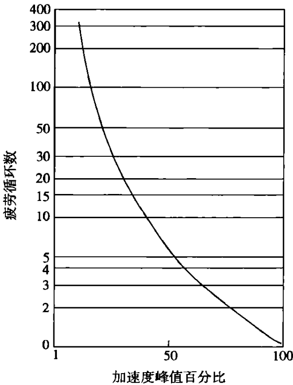
图 8 地震动循环次数的确定
