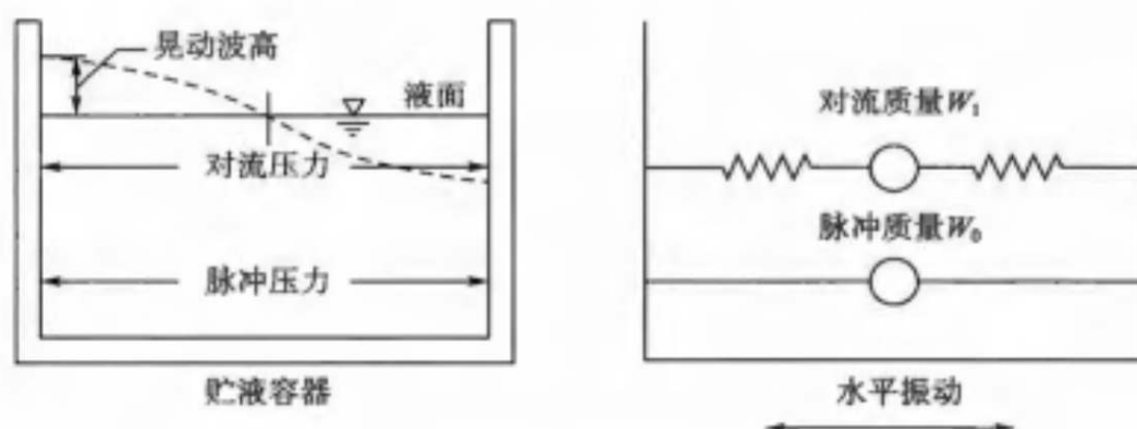
图 4 贮液容器中动液压效应示意图
