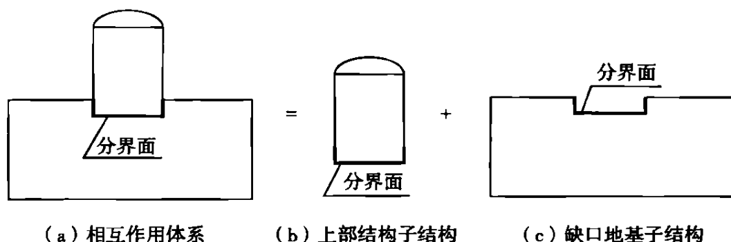
图 A.3.1 相互作用体系模型示意图
