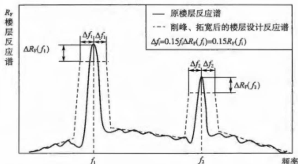
图 D.0.1 反应谱的削峰和拓宽
