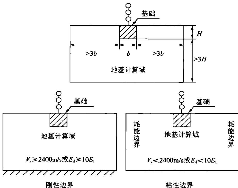
图 A.2.1 地基有限元计算域
