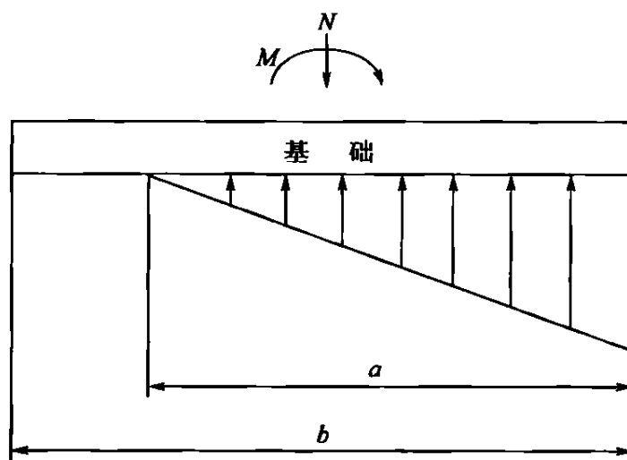
图 5.2.6 矩形基础底面接地率计算
