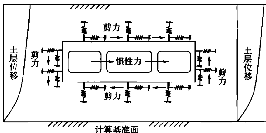
图 J.1.1 反应位移法计算模型示意图
