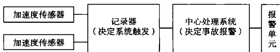
图 7 核电厂地震监测与报警系统示意图
