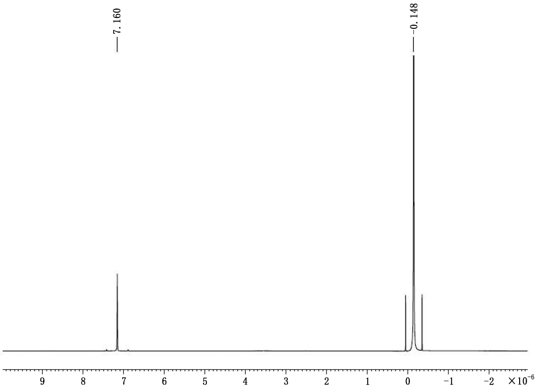
图 A.1 三甲基镓典型核磁谱图
