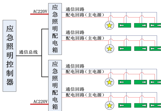
图 17 应急照明控制器与应急照明配电箱之间采用树形通信总线的集中控制型系统
