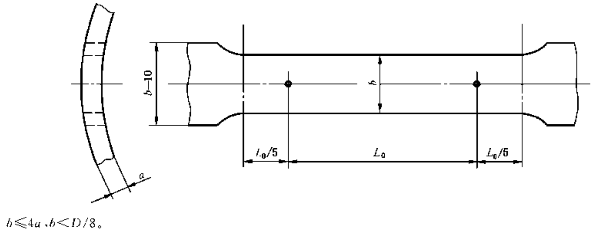
图 5 拉伸试样图
