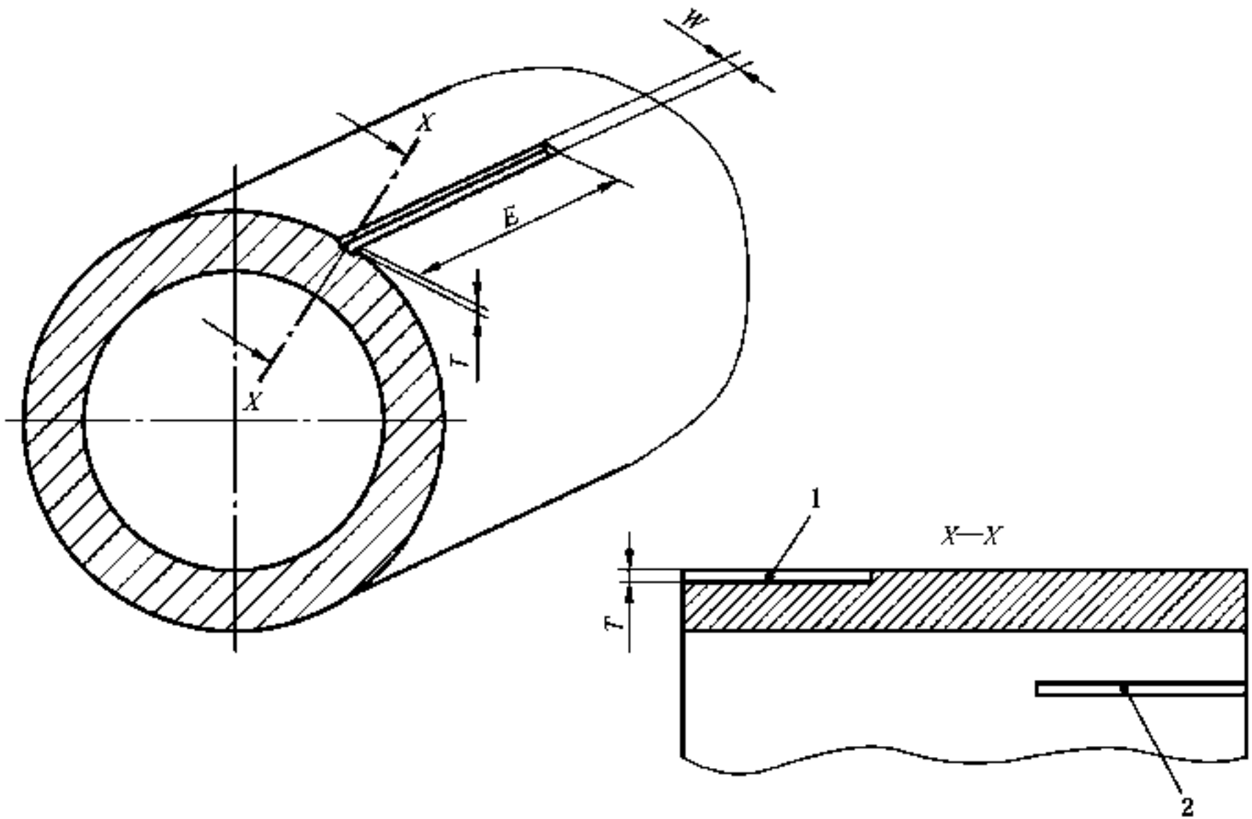
图 B.1 筒体/瓶底过渡区
