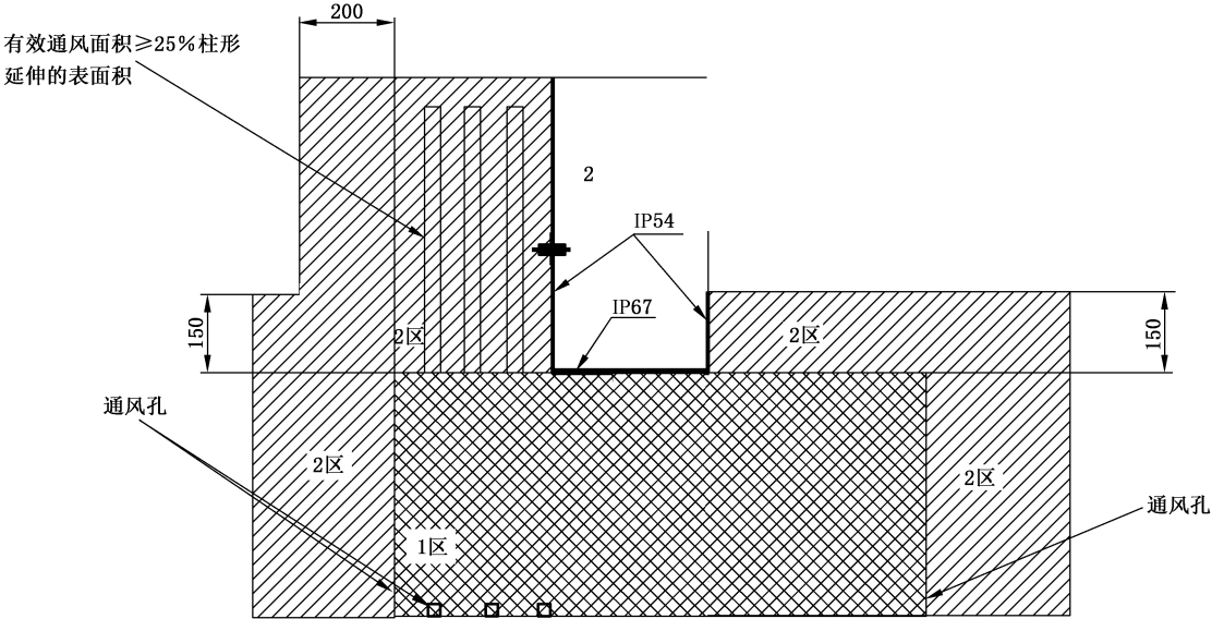
a) 油气屏障为 1 型
