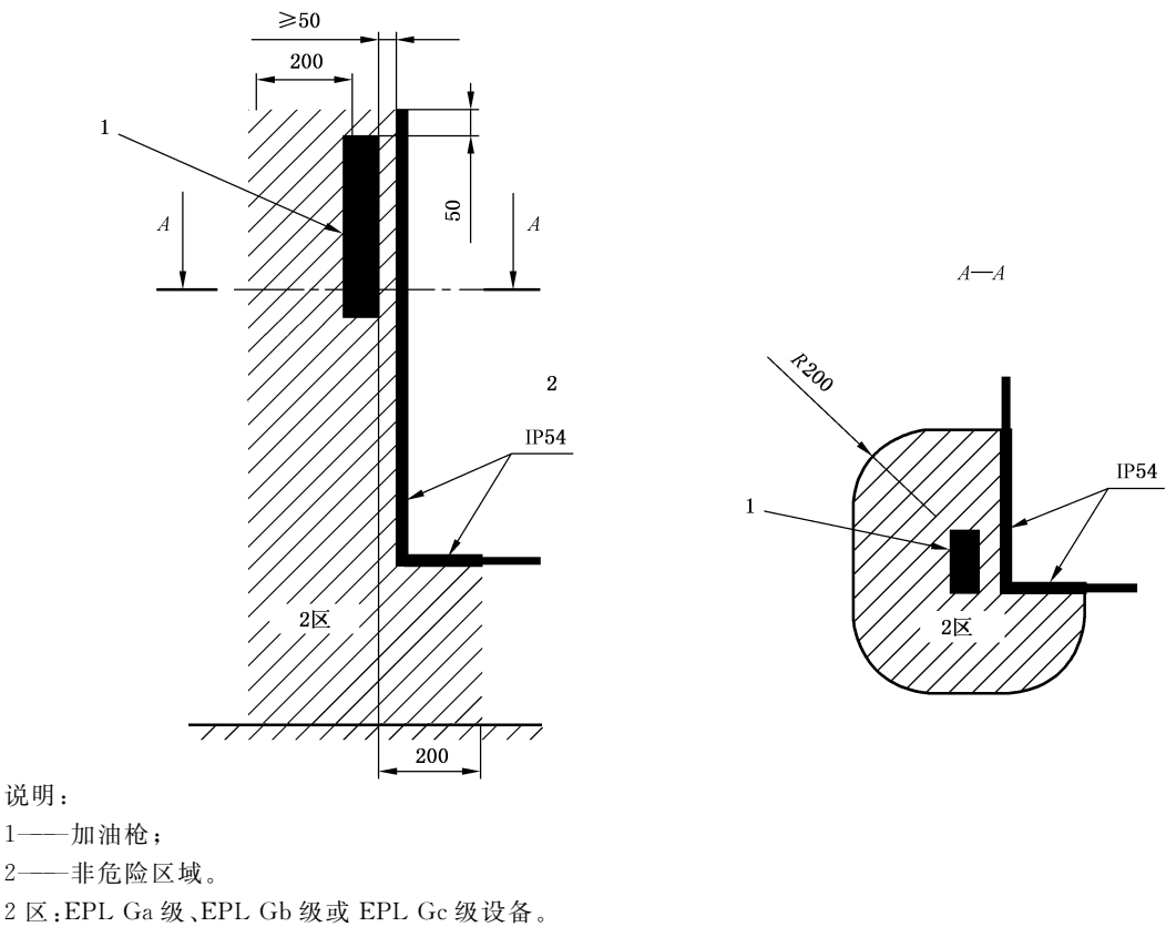
图 1 加油枪位置在外壳外部(50 mm<与外壳间距≤200 mm)
