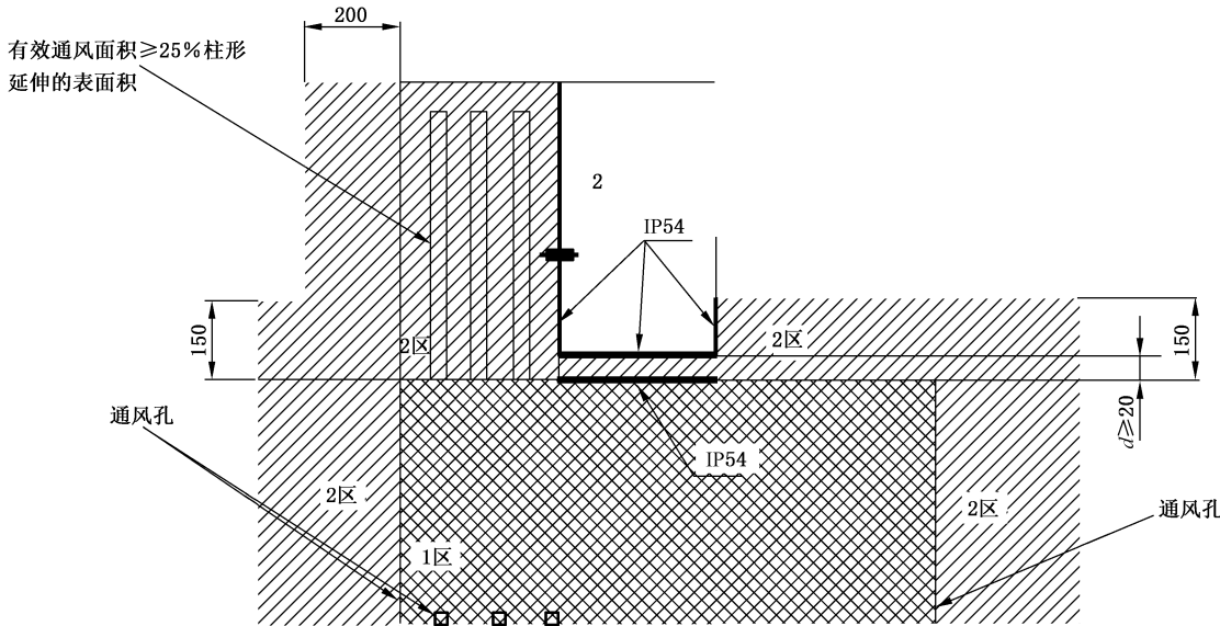
b) 油气屏障为 2 型
