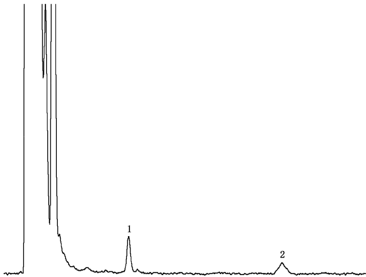
图 2 六氯苯、十氯联苯标样的高效液相色谱图
