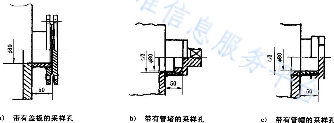
图 A.2 几种封闭形式的采样孔
