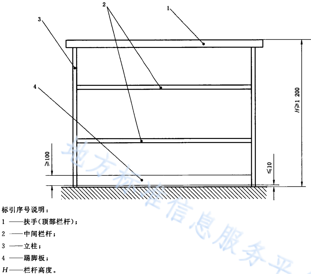
图 A.6 防护栏杆示意图
