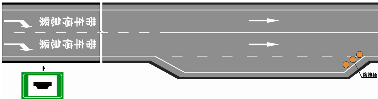
图26 隧道紧急停车带安全设施设置示例
