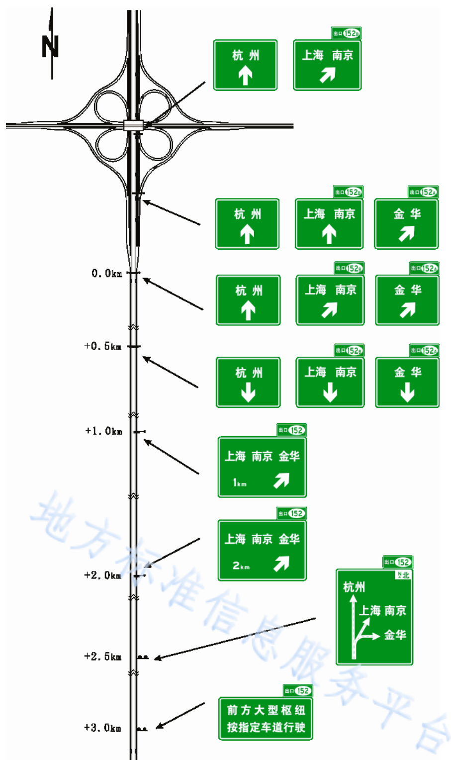
图C.4 苜蓿叶形互通交通标志布置示例(带集散车道)
