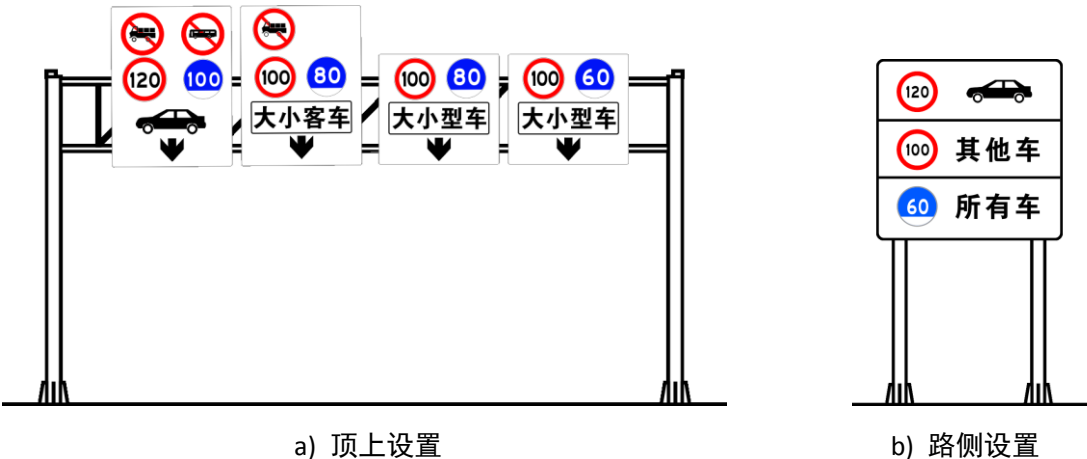
图18 限制速度的设置方式示例
