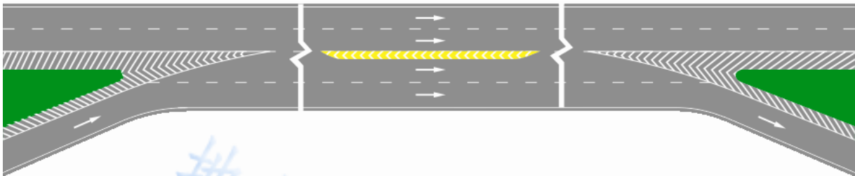
图34 复合式路段标线一般渠化示例
