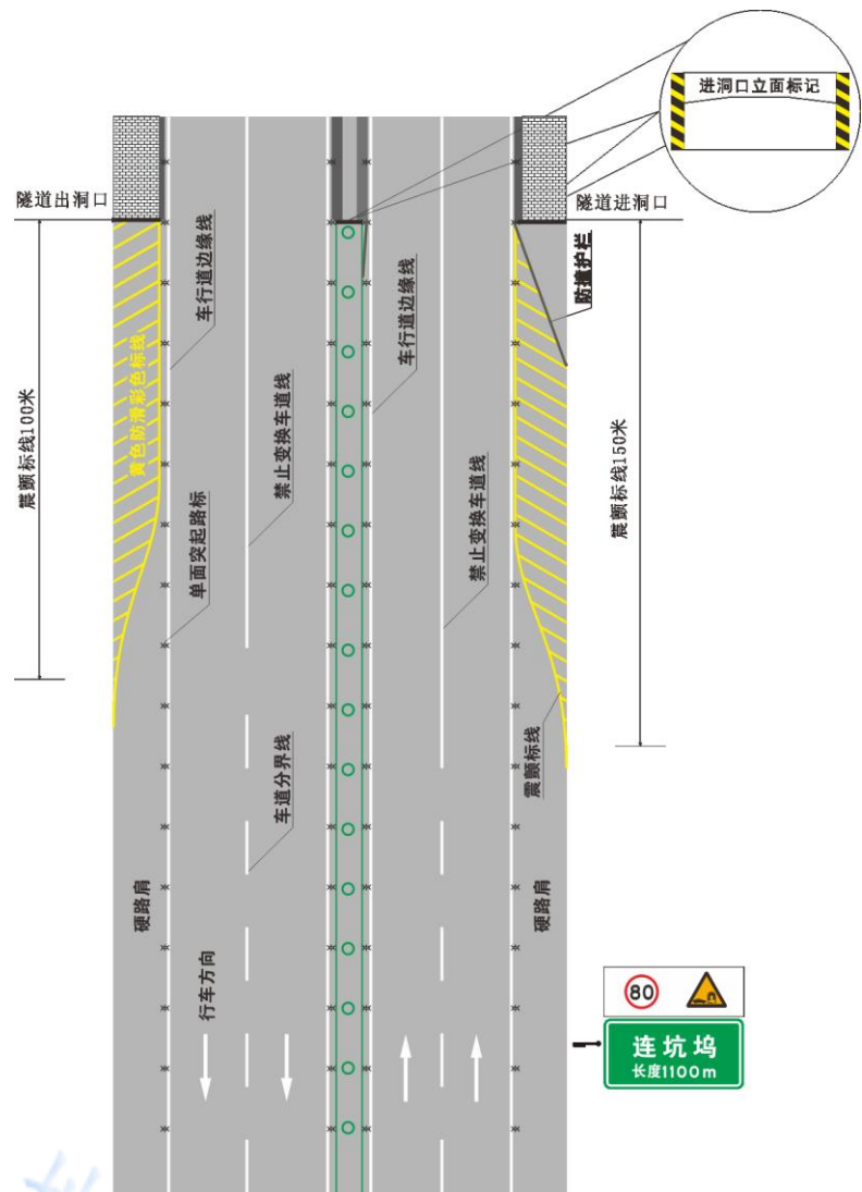
图25 隧道入口视觉过渡措施示例
