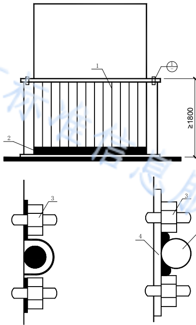
1-钢筋铁栅门 2-踢脚板 3-M12 膨胀螺栓 4-10 厚钢板 5- \Phi 48.3 \times 3.6 mm 钢管
