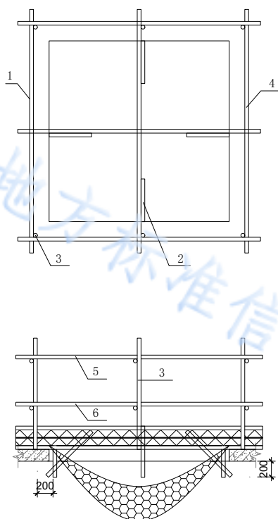
图 5.2.9-1 边长 1500-2000mm 的洞口防护
