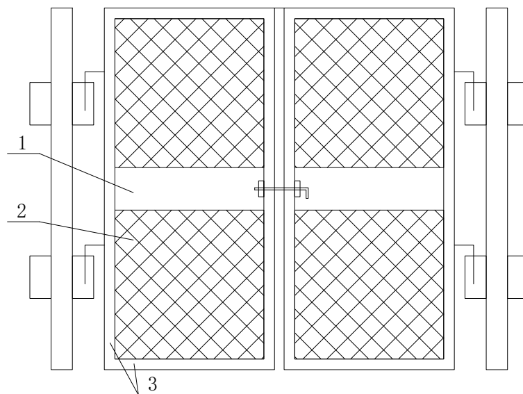
1-150 宽 3 厚钢板 2-钢丝网片 3-40x4 方管
