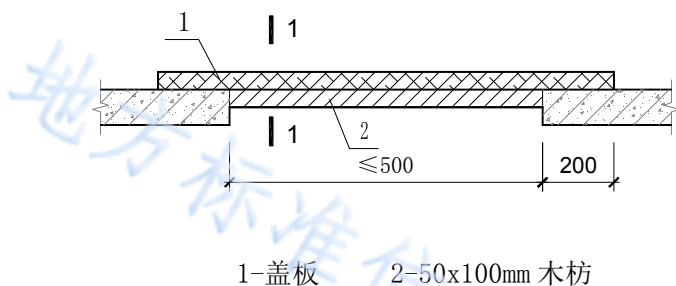
图 5.2.1-1 洞口盖板防护平面图
