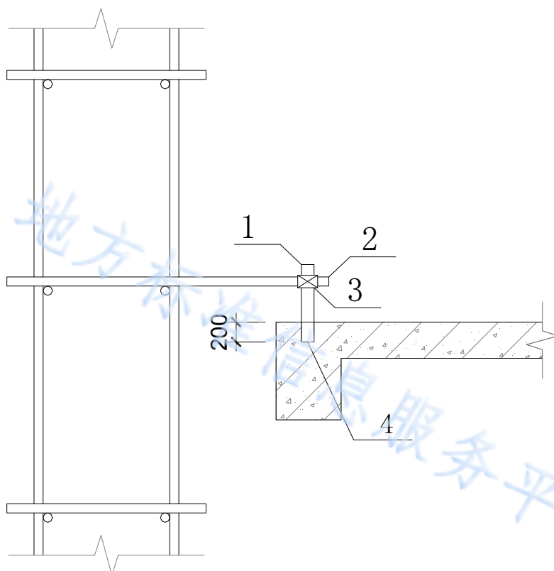
1-预埋短钢管 2-连墙件 3-扣件 4-结构梁
