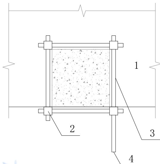
图 8.4.8-3 钢管扣件刚性连墙杆示意图 (一)
