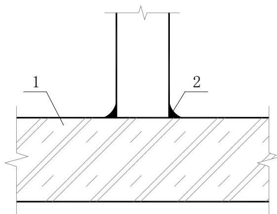
图 4.8.2-2 装配式工程梁面临时护栏示意图 (二)
