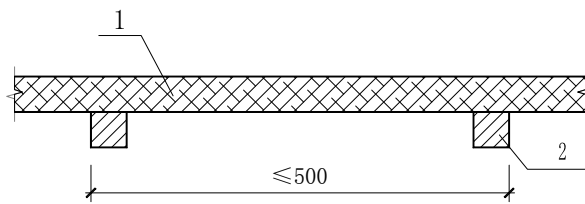
1-盖板 2-50x100mm 木枋
