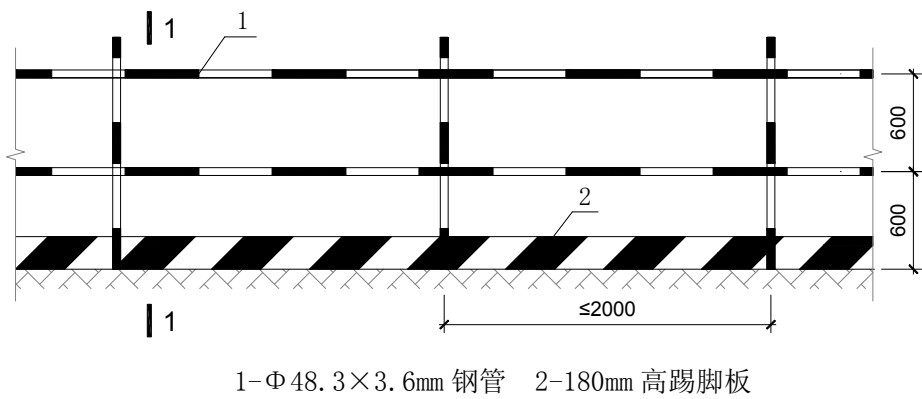
图 4.5.3-1 基坑周边防护立面图
