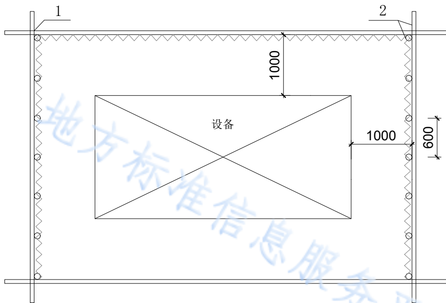
图 7.3.5-1 设备安全防护棚立面图
