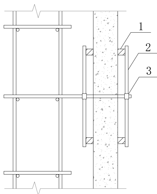
1-垫木 2-短钢管 3-直角扣件
