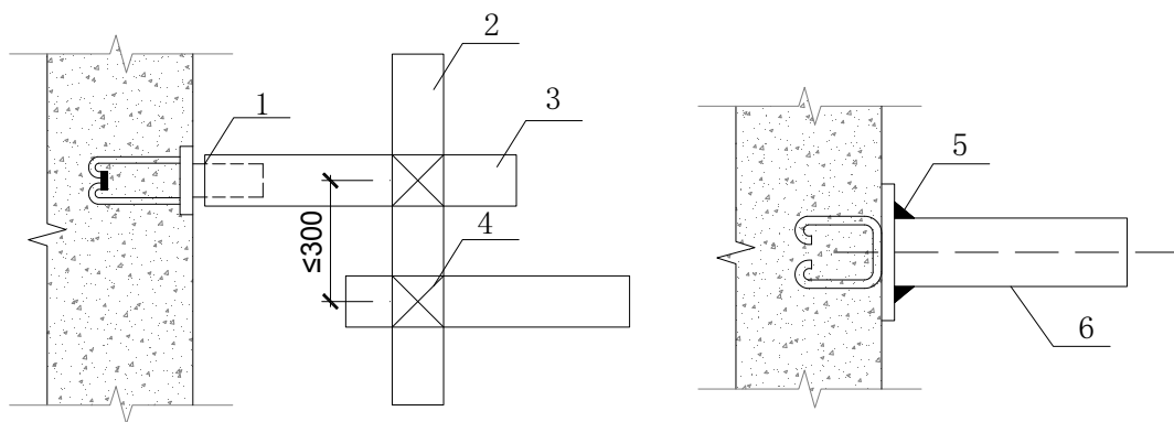
图 8.4.8-2 钢管焊接刚性连墙杆示意图
