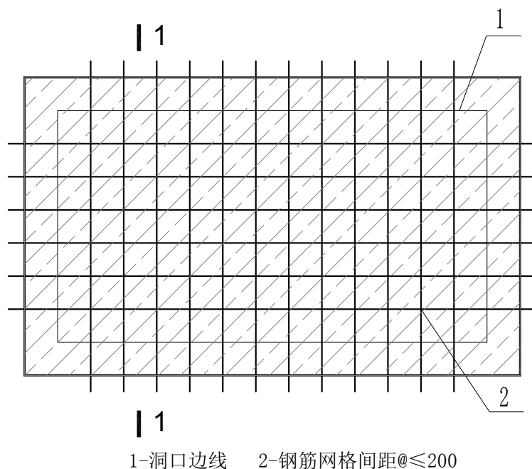
图 5.2.7-1 边长小于 1500mm 的洞口钢筋防护平面图
