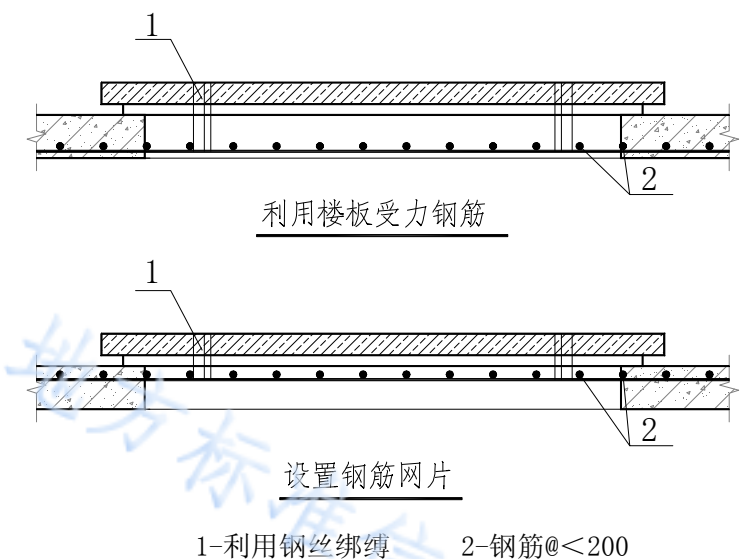
图 5.2.7-2 边长小于 1500mm 的洞口钢筋防护 1-1 剖面图
