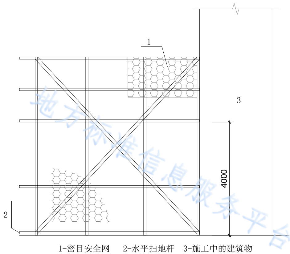
图 7.3.3-2 施工电梯、物料提升机地面进料口安全通道侧面图
