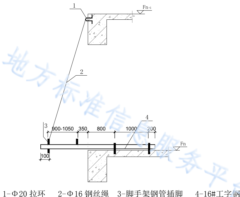
图 8.2.5-1 框架部位或剪力墙上开孔时侧面示意图
