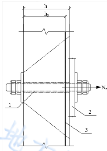
图 4.2.3-2 附着螺栓孔处混凝土受冲切状况图
