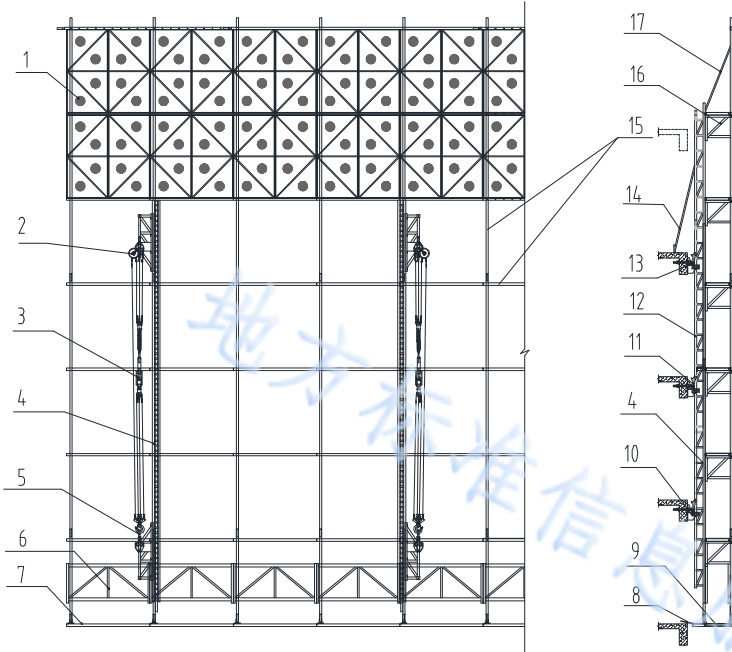
图 5.1.1 附着式升降脚手架构造示意图
