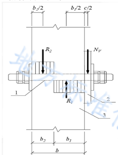
图 4.2.3-1 附着螺栓孔处混凝土受压状况图
