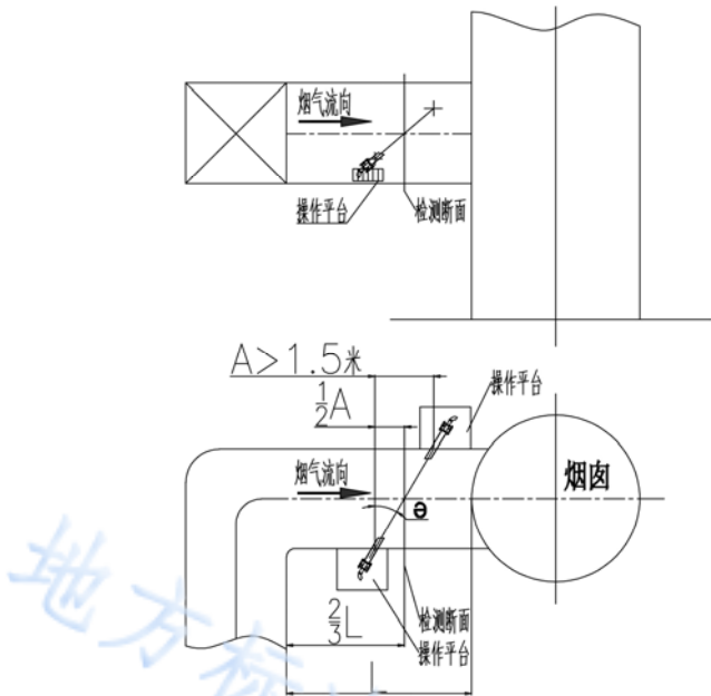
图 B.1 超声波气体流速计单条安装示意图
