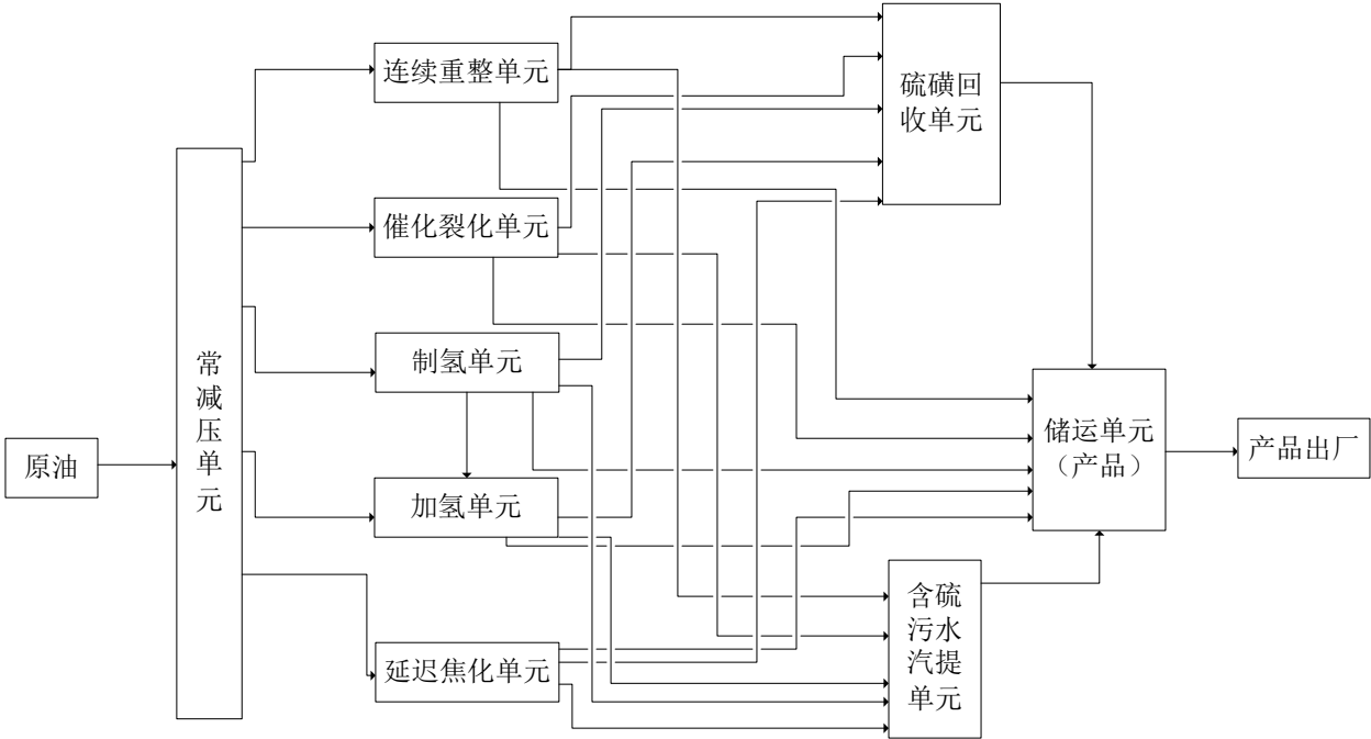
图B.1 原油加工企业典型工艺流程示意图
