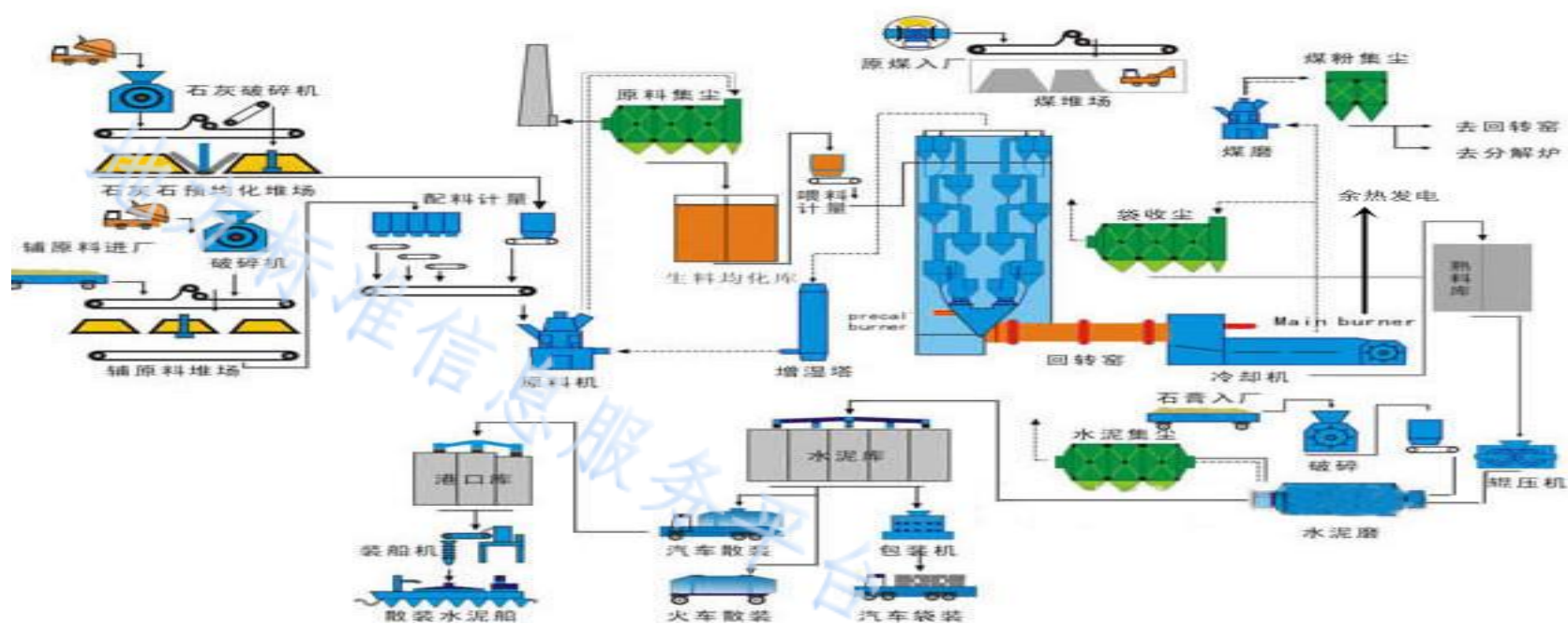
图B.1 水泥制造企业典型工艺流程图
