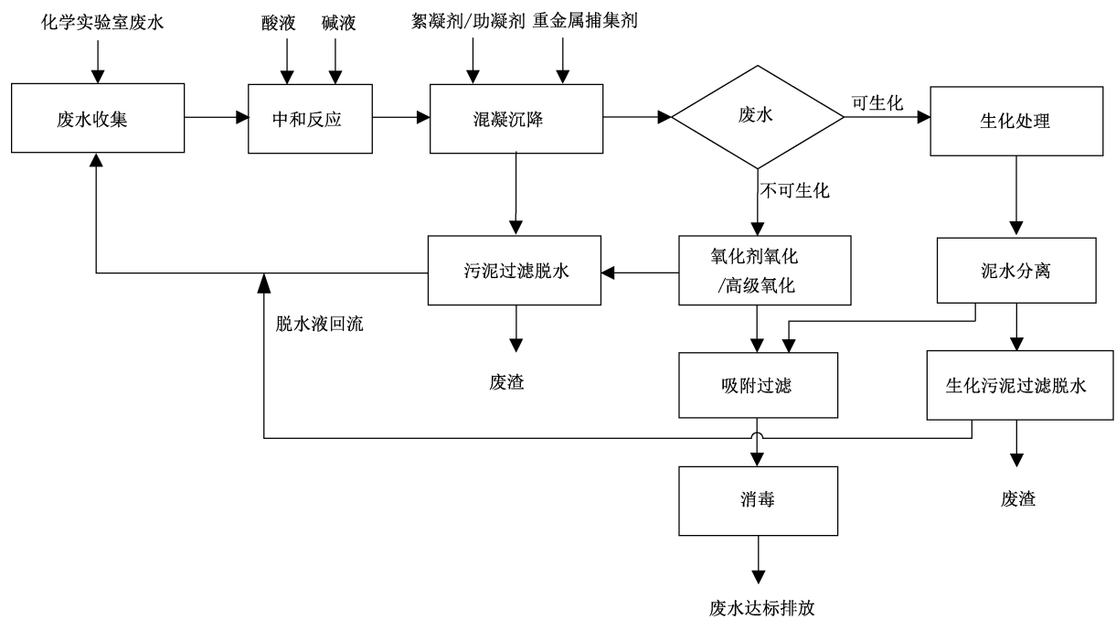
图 1 化学实验室废水处理工艺流程
