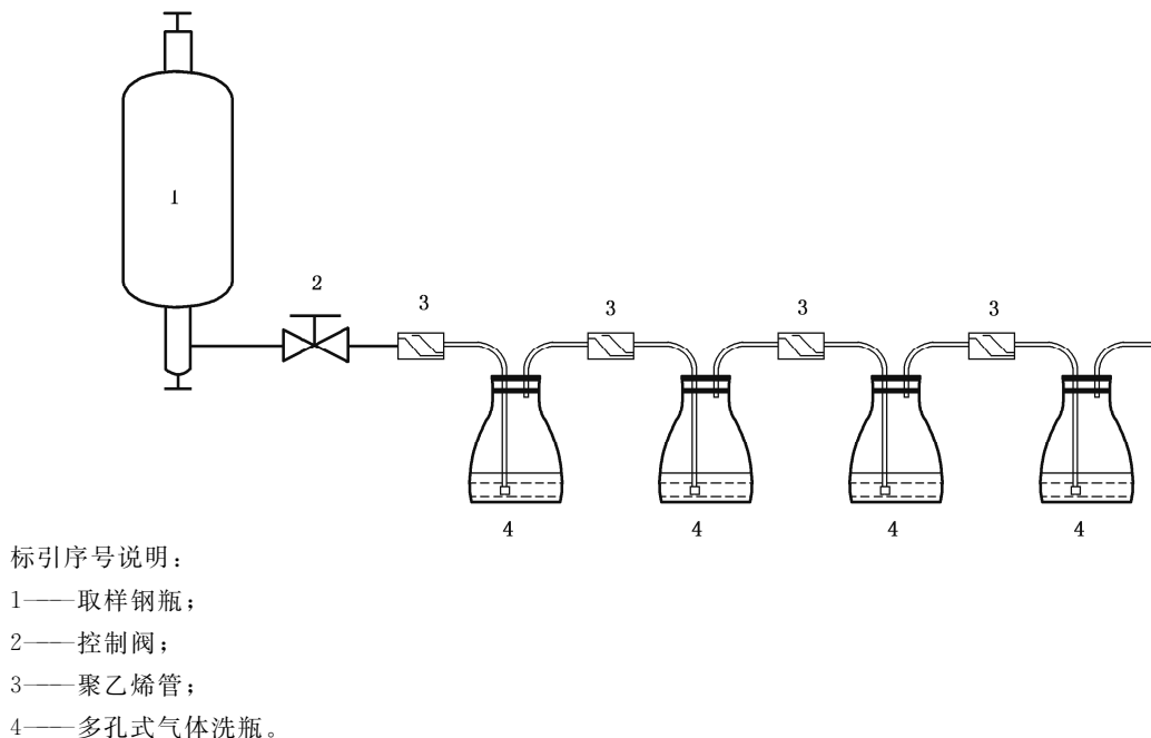
图 1 酸度测定装置示意图
