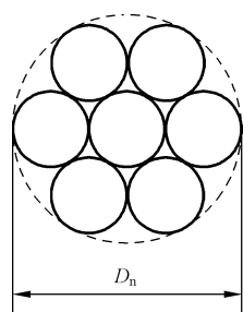
图 1 1×7 钢绞线横截面外形示意图
