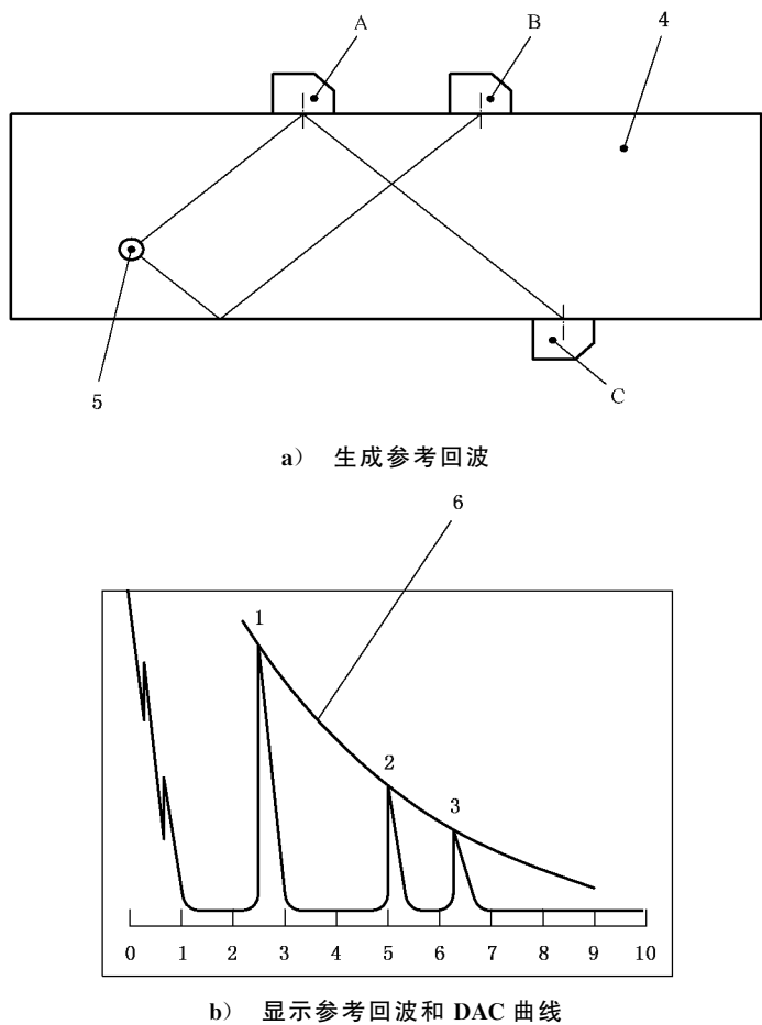
说明： 1——位置 A 的参考回波； 2——位置 B 的参考回波； 3——位置 C 的参考回波； 4——对比试块； 5——参考反射体； 6——距离幅度曲线(DAC)。
