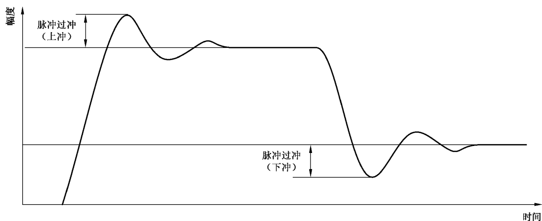
图 3 脉冲过冲
