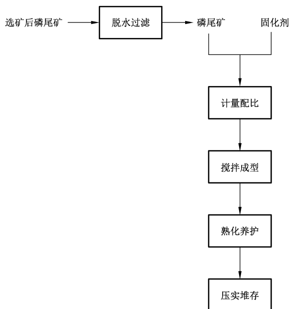
图 3 固化处理法工艺流程图
