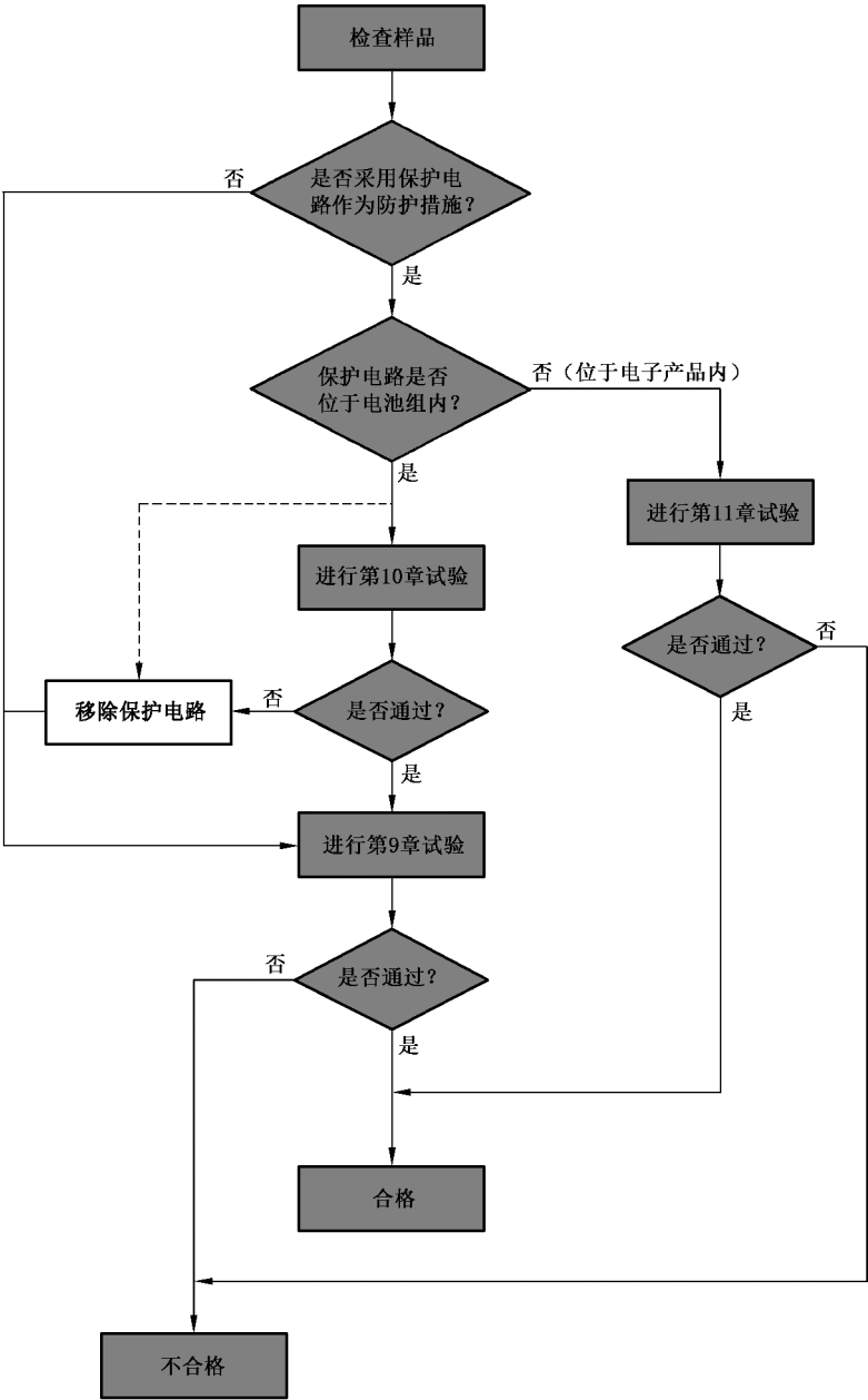
图 B.3 电池组电安全试验顺序
