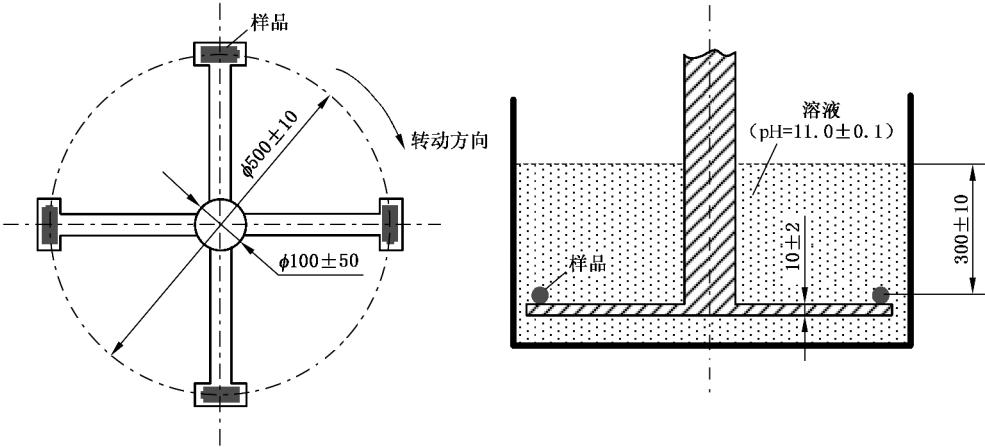
图 C.3 洗涤试验装置
