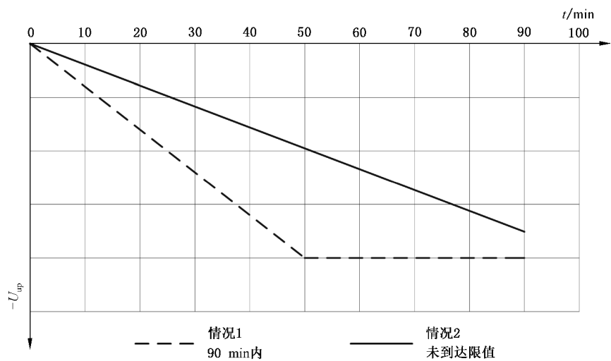
图 2 强制放电示意图
