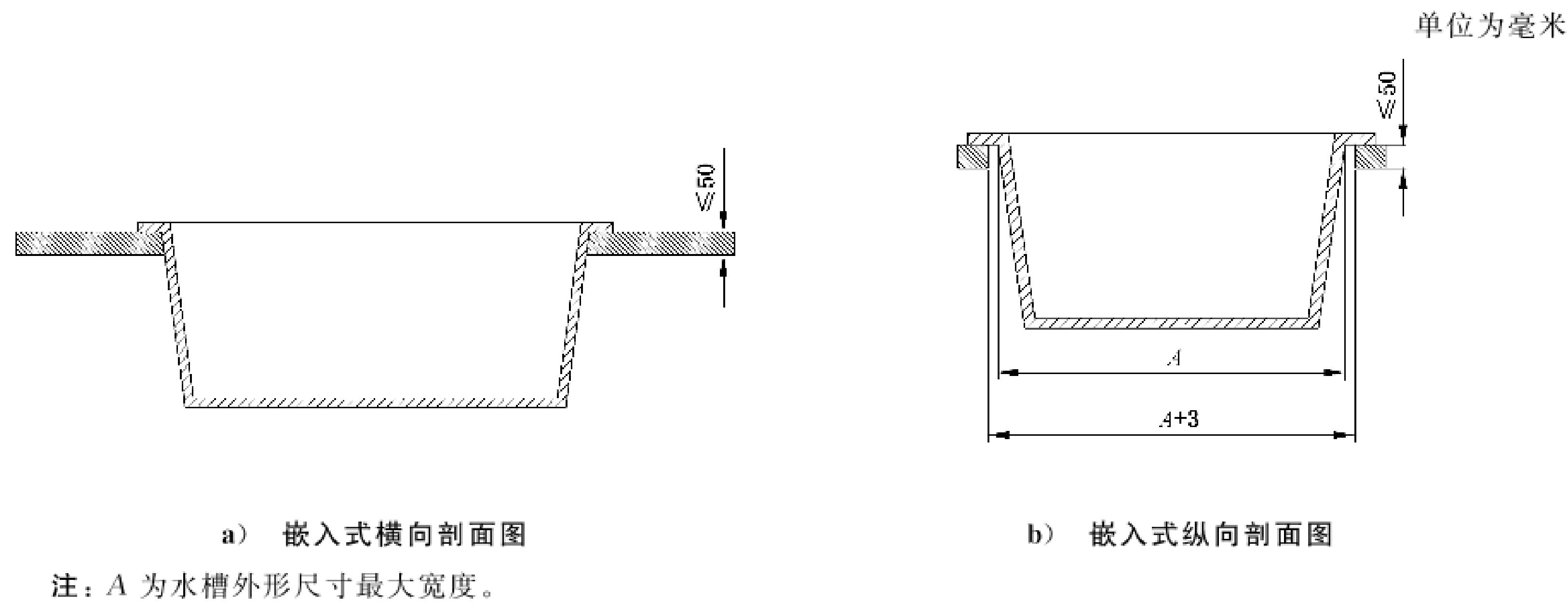
图 1 嵌入式安装
