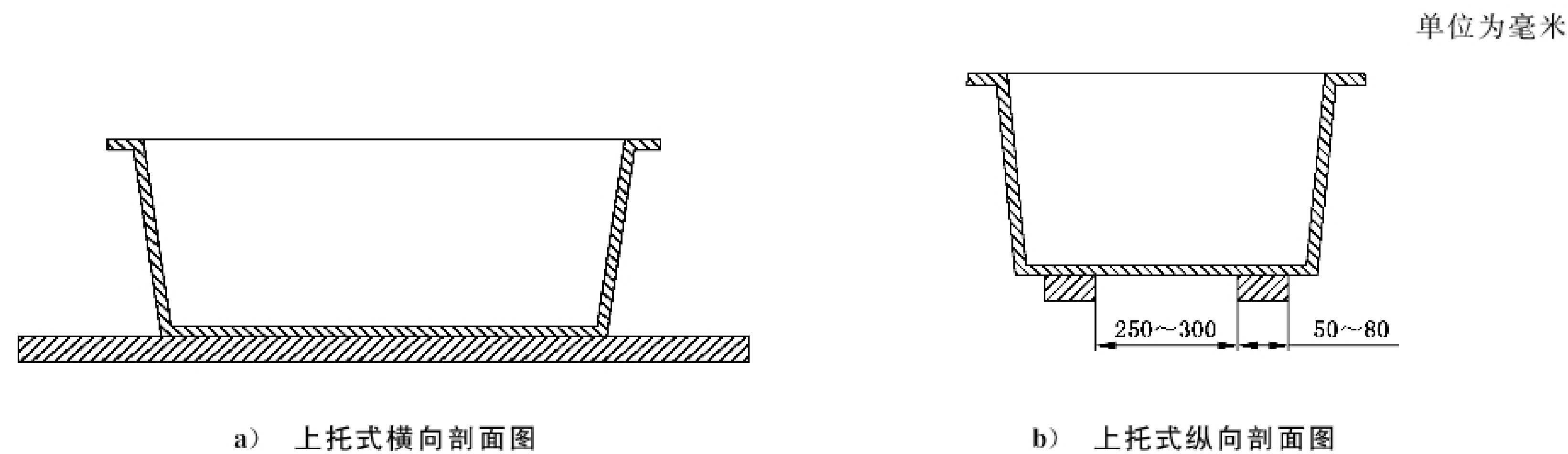
图 2 上托式安装
