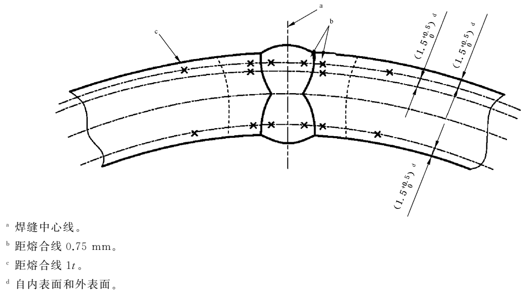
图 1 SAW 管硬度试验位置
