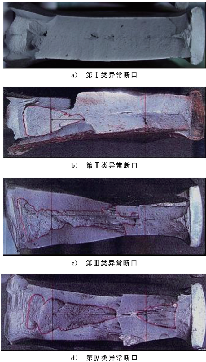
图 B.2 异常断口分类
