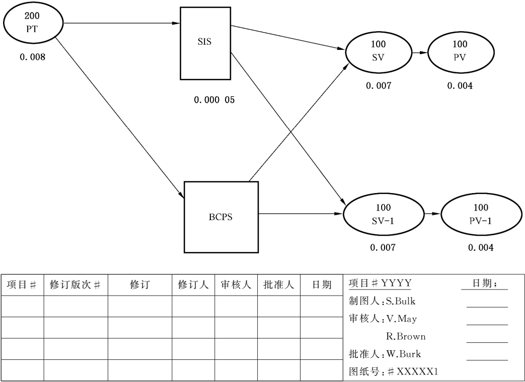
图 F.8 显示每个 SIS 设备 PFD_{avg} 的 SIF S-3 气泡图
