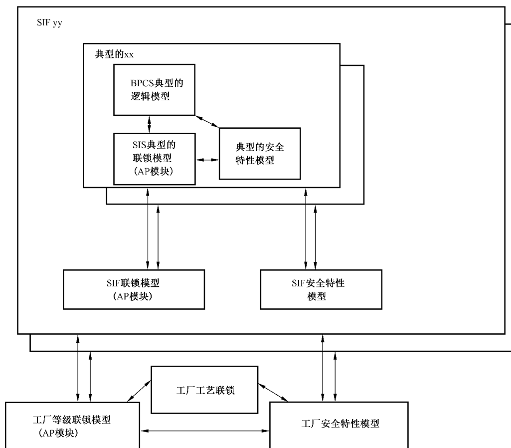
图 B.10 包括安全特性模型和 BPCS 逻辑模型的模型集成的层级结构
