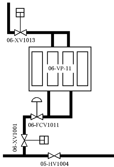
图 B.2 SIF 06.02 工艺流程图
