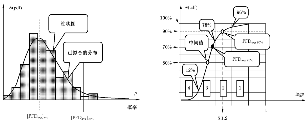
图 A.7 根据蒙特卡罗模拟得出的目标结果的典型概率分布
