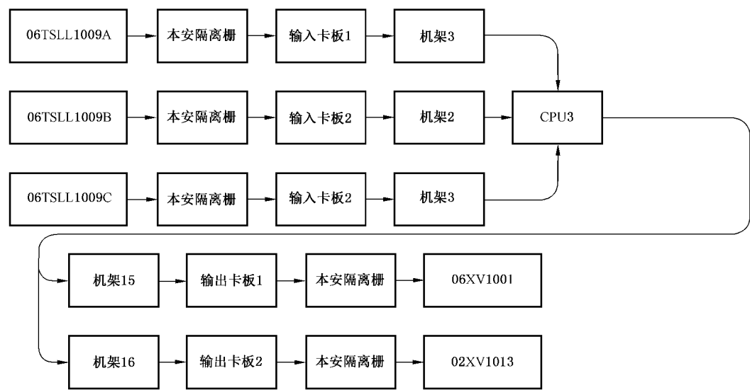
图 B.8 SIF 06.02 硬件物理架构
