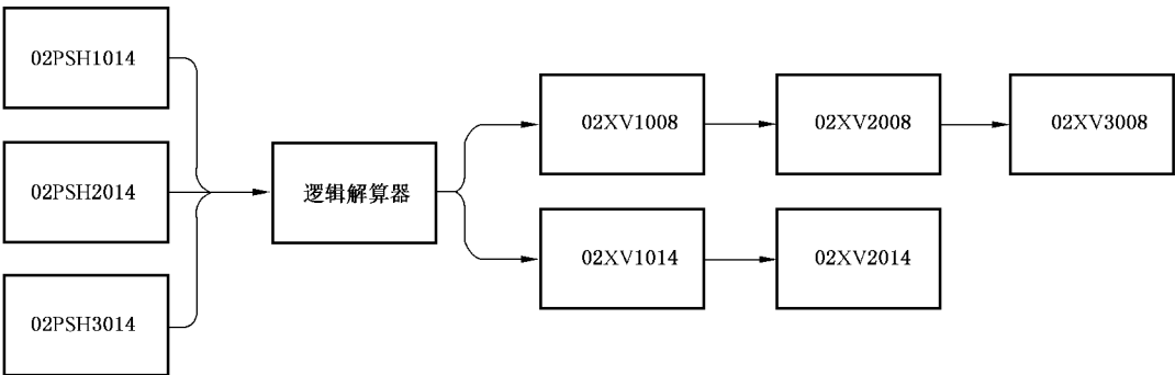
图 B.4 SIF 02.01 硬件功能架构
