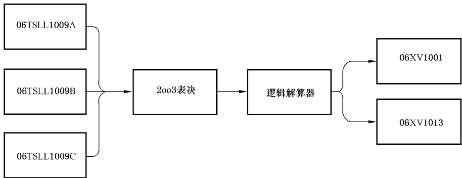
图 B.5 SIF 06.02 硬件功能架构
