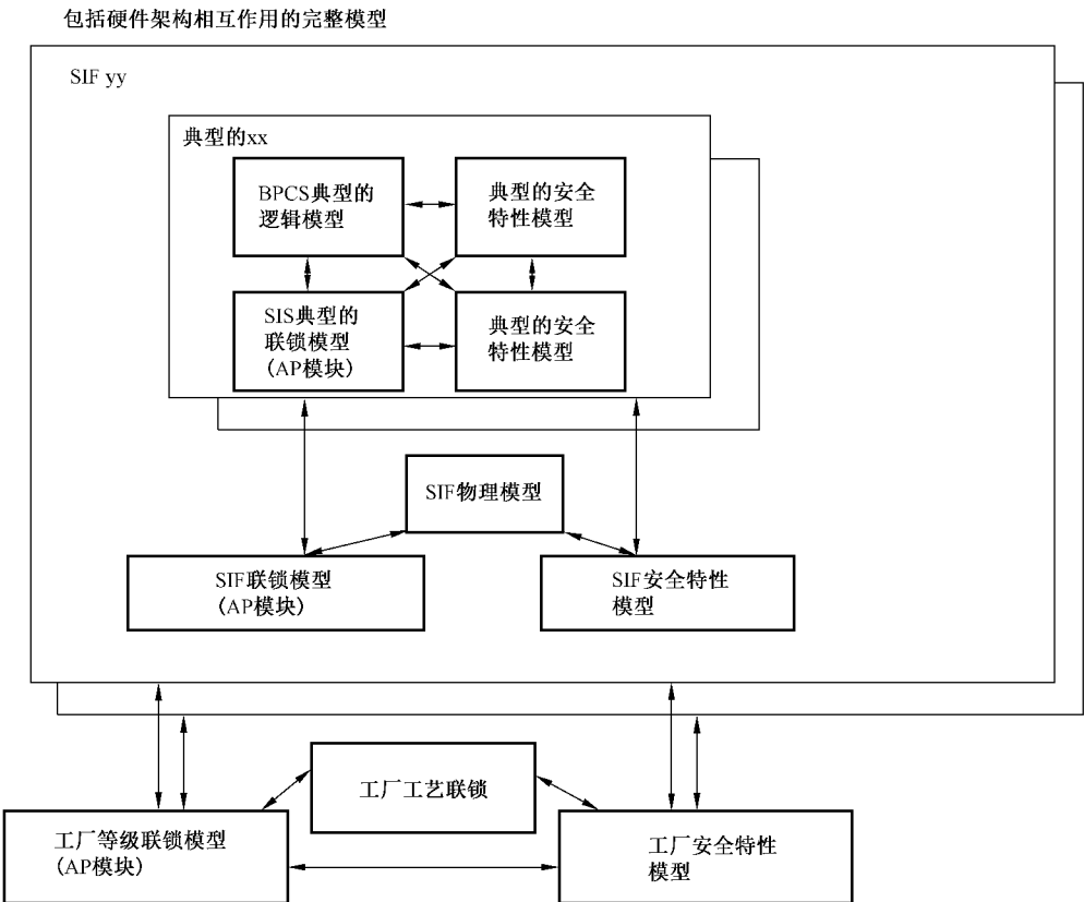
图 B.16 用于最终实现模型检查的完整模型
