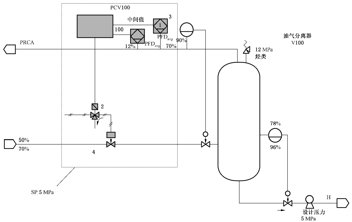
图 D.1 油气分离器的 P&ID 示例
