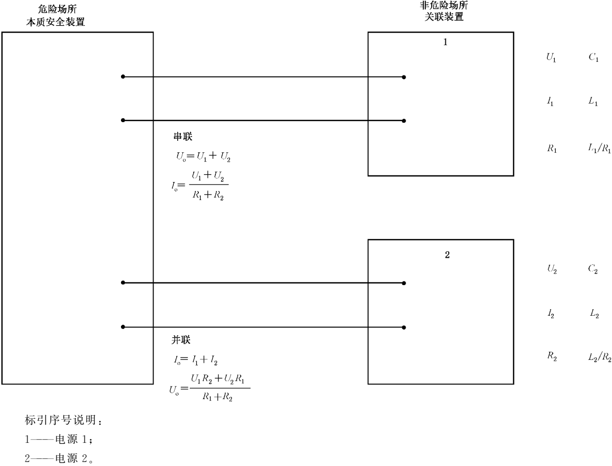
图 E.3 非预期连接的电源
