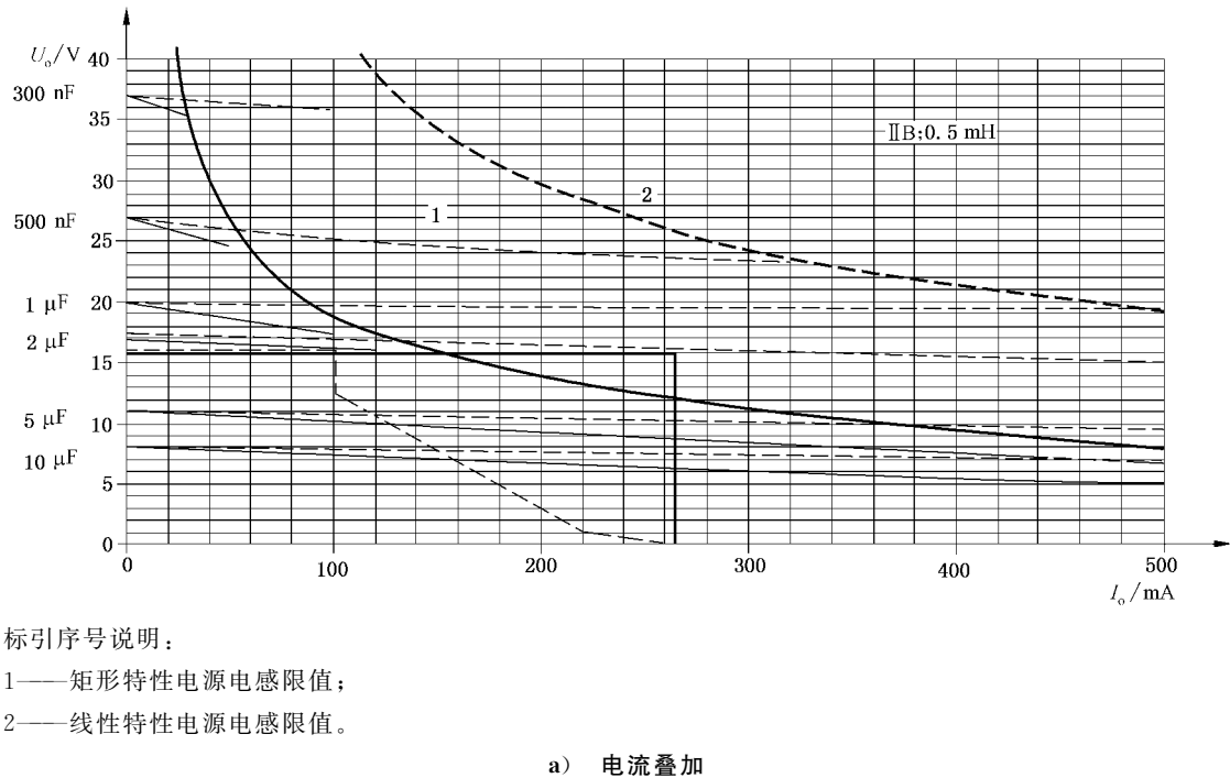
图 F.6 图 F.4 所给示例的电流叠加和/或电压叠加
