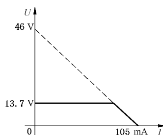
a) 输出特性
