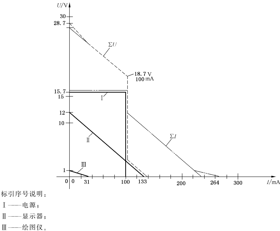
图 F.5 图 F.4 所给电路的总特性
