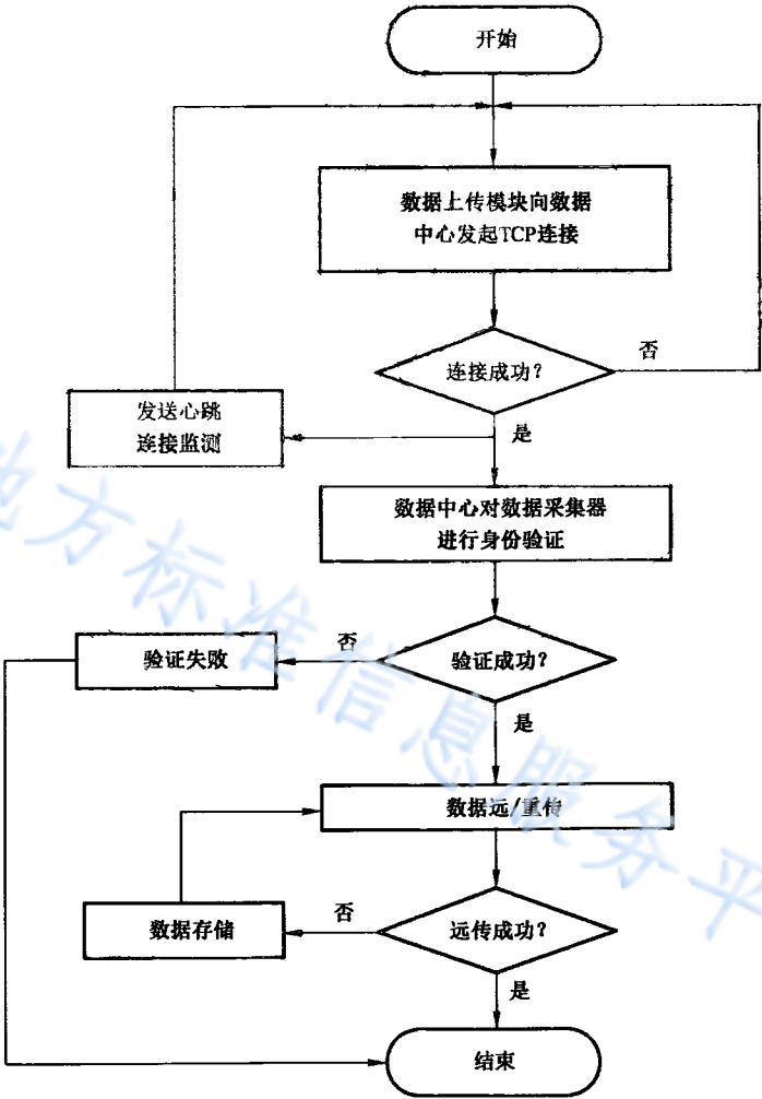
图 C.1 通信流程图
