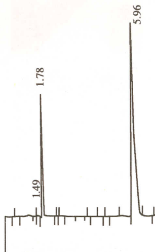
图 1 色谱分离图
